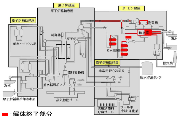
系統概略図
