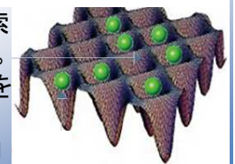
光格子の模式図
