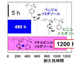
アルカリ水、80°Cでの耐久性
