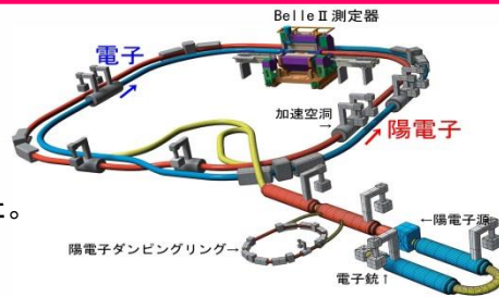
SuperKEKB(周長約3km)
