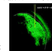
蛍光寿命二光子励起レーザー顕微鏡で測定した微小領域内での化学反応
