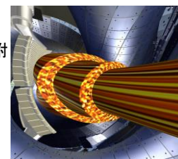
◆大型ヘリカル装置のプラズマ中の乱流をスーパーコンピュータを用いてシミュレート (予測研究)
