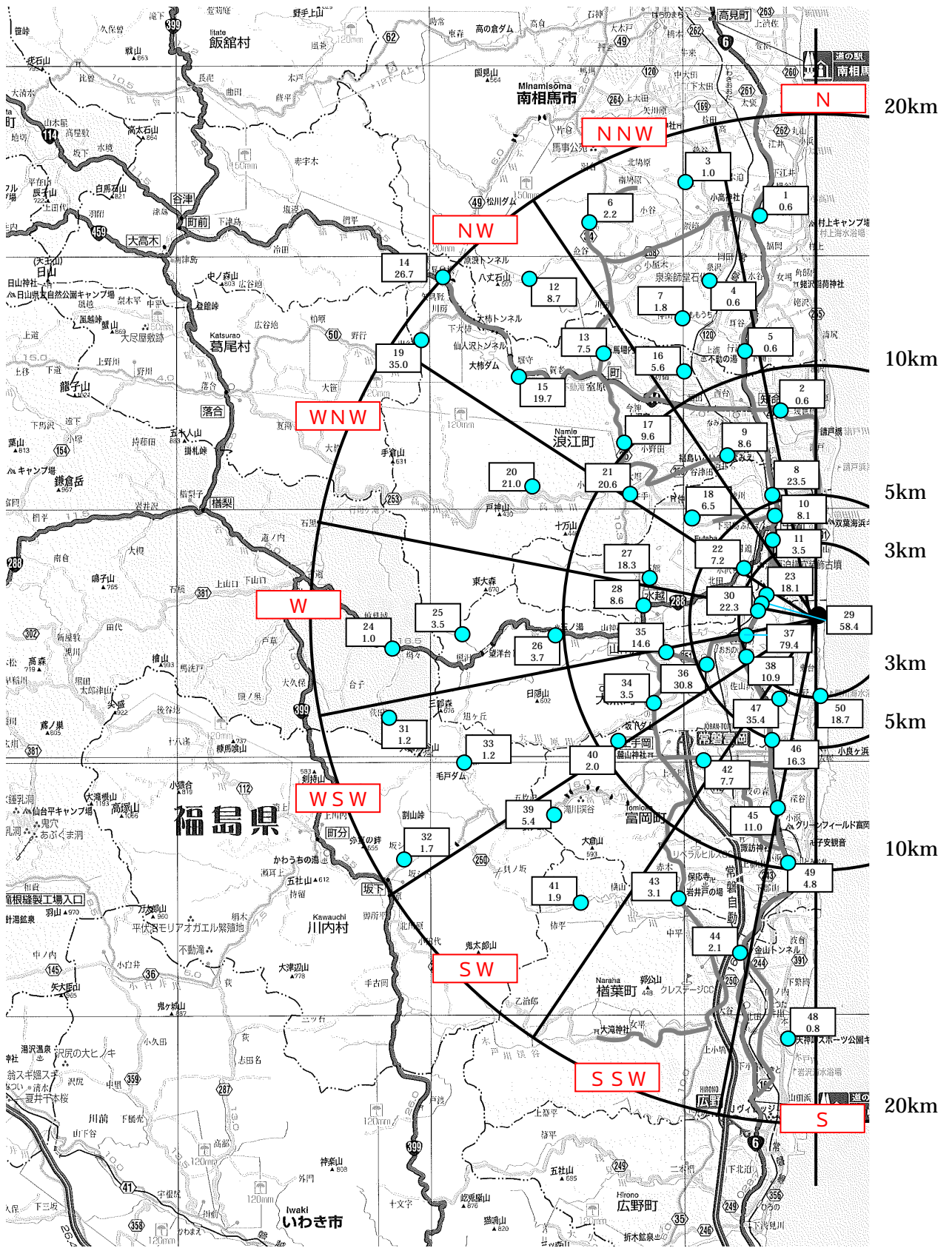
福島第一原子力発電所より 20km 圏内の空間放射線量率測定結果 (測定日:平成 23 年 7 月 2 9 日)
