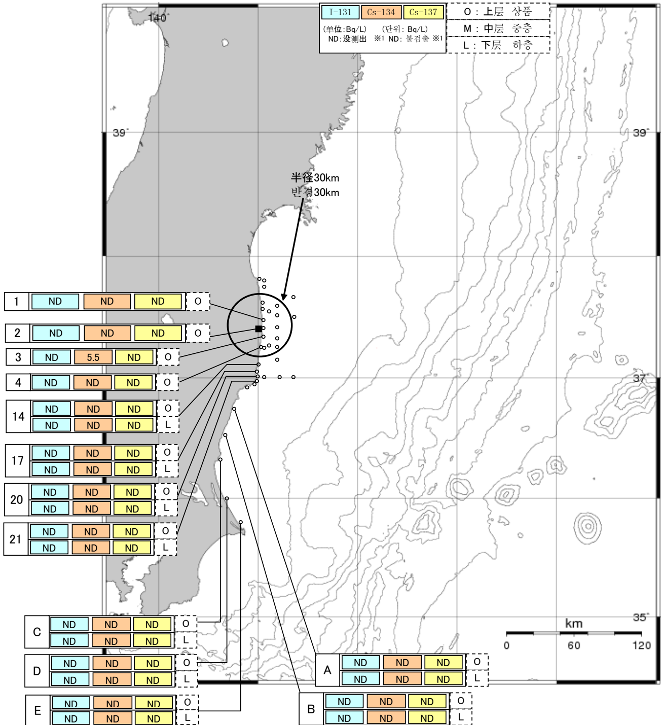
图中■表示东京电力福岛第一核电站 도표 안의 ■은 도쿄전력 후쿠시마 제1원자력발전소를 나타냄 *文部科学省根据东京电力报告编制 ( http://www.tepco.co.jp/cc/press/index11-j.html ) 문부과학성이 도쿄전력의 보고에 의거해 작성. ( http://www.tepco.co.jp/cc/press/index11-j.html ) ※1 ND表示海水核辐射含量的检测值低于检测极限值(东京电力福岛第一核电站周边, 碘131约为9Bq/L, 铯134约为23Bq/L, 铯137约为25Bq/L。茨城县沿岸, 碘131约为7Bq/L, 铯134约为17Bq/L, 铯137约为16Bq/L)。 ※1 ND의 기재는 해수 방사능 농도의 검출치가 검출 한계치(도쿄전력 후쿠시마 제1원자력발전소 주변에 대해서는 I-131이 약 9Bq/L, Cs-134가 약 23Bq/L 및 Cs-137이 약 25Bq/L, 이바라키현 연안에 대해서는 I-131이 약 7Bq/L, Cs-134가 약 17Bq/L 및 Cs-137이 약 16Bq/L)를 밑도는 경우.
