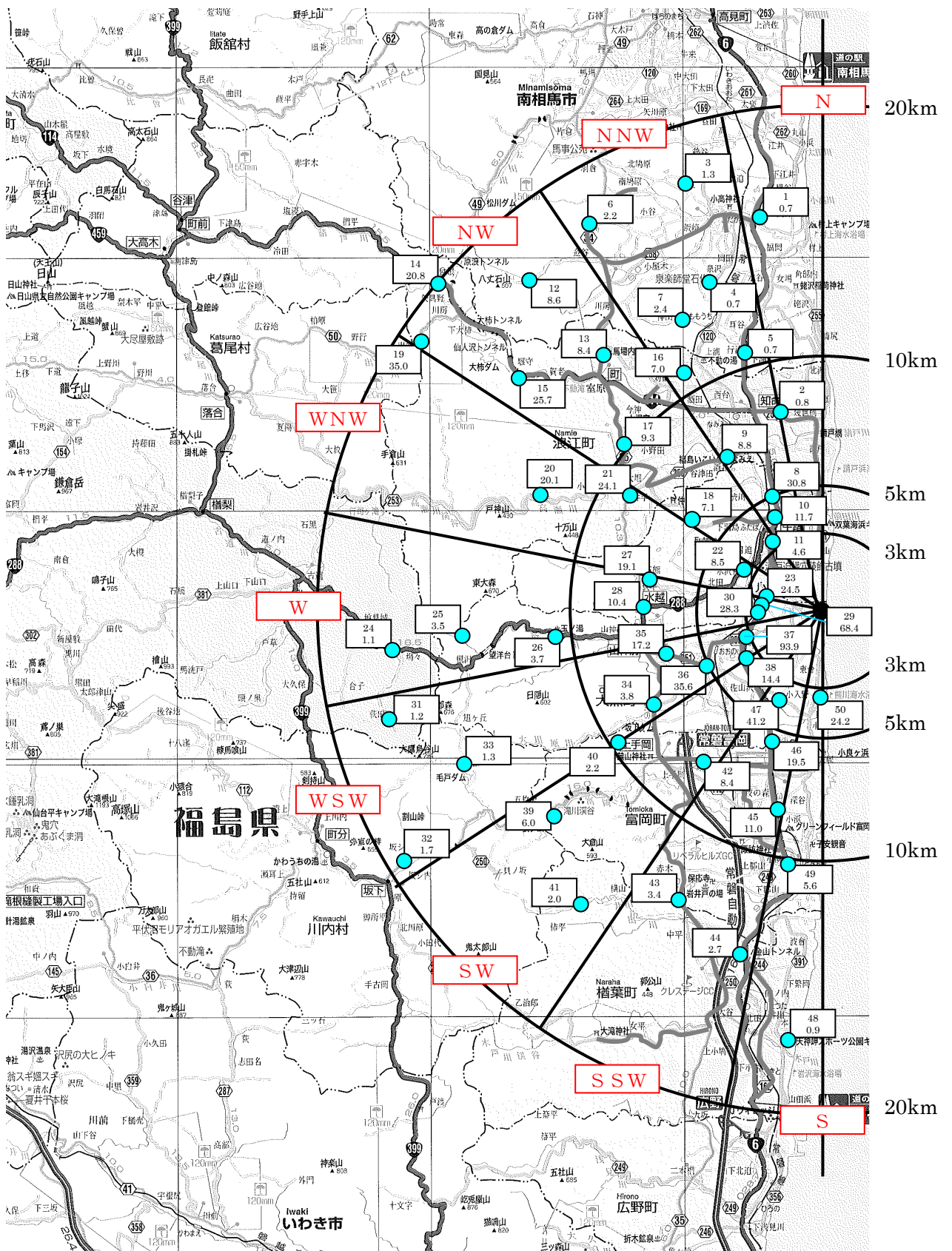
福島第一原子力発電所より 20km 圏内の空間放射線量率測定結果 (測定日：平成 23 年 6 月 3 日)
