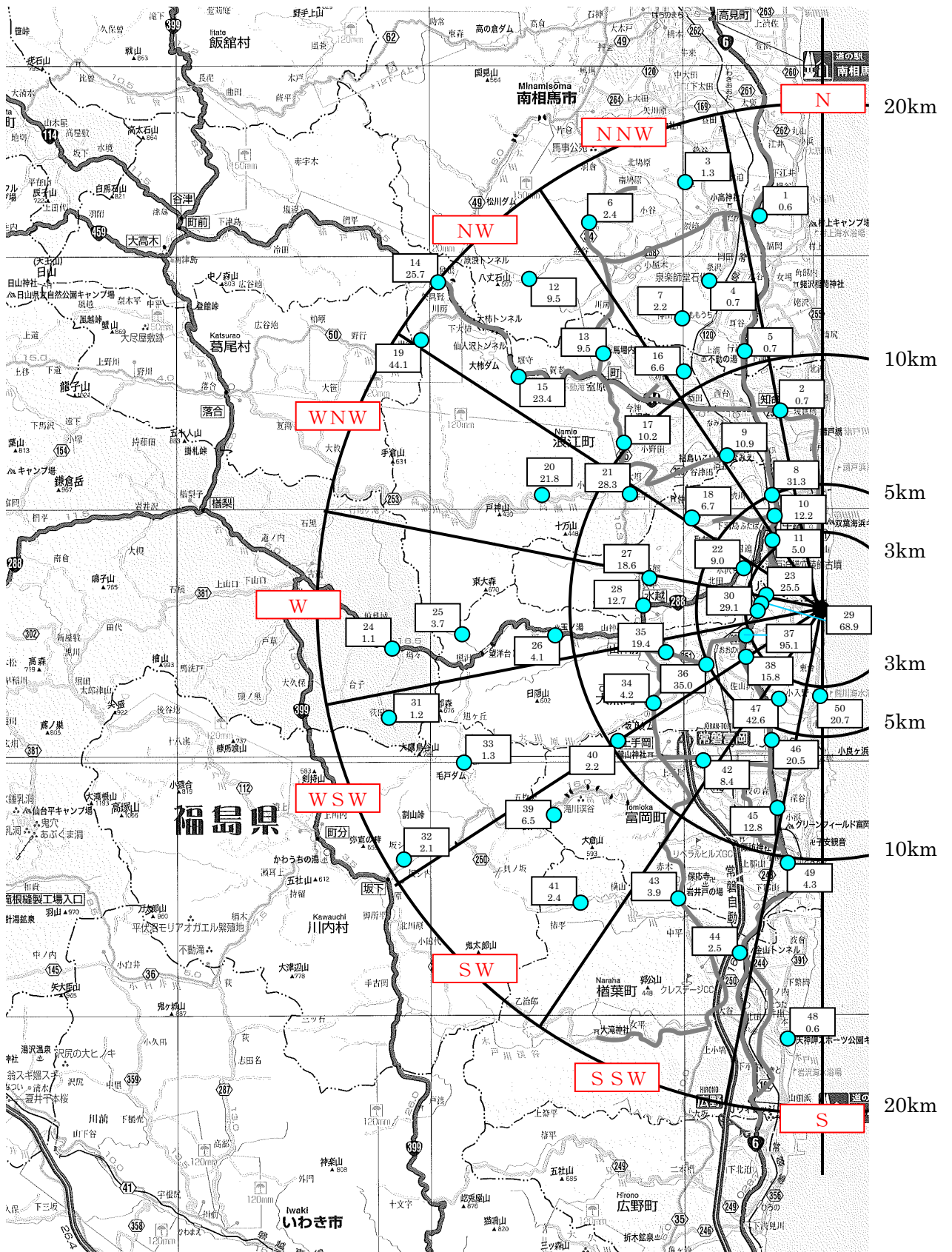
후쿠시마 제 1 원자력발전소에서 20km 권내의 공간 방사선량을 측정 결과
