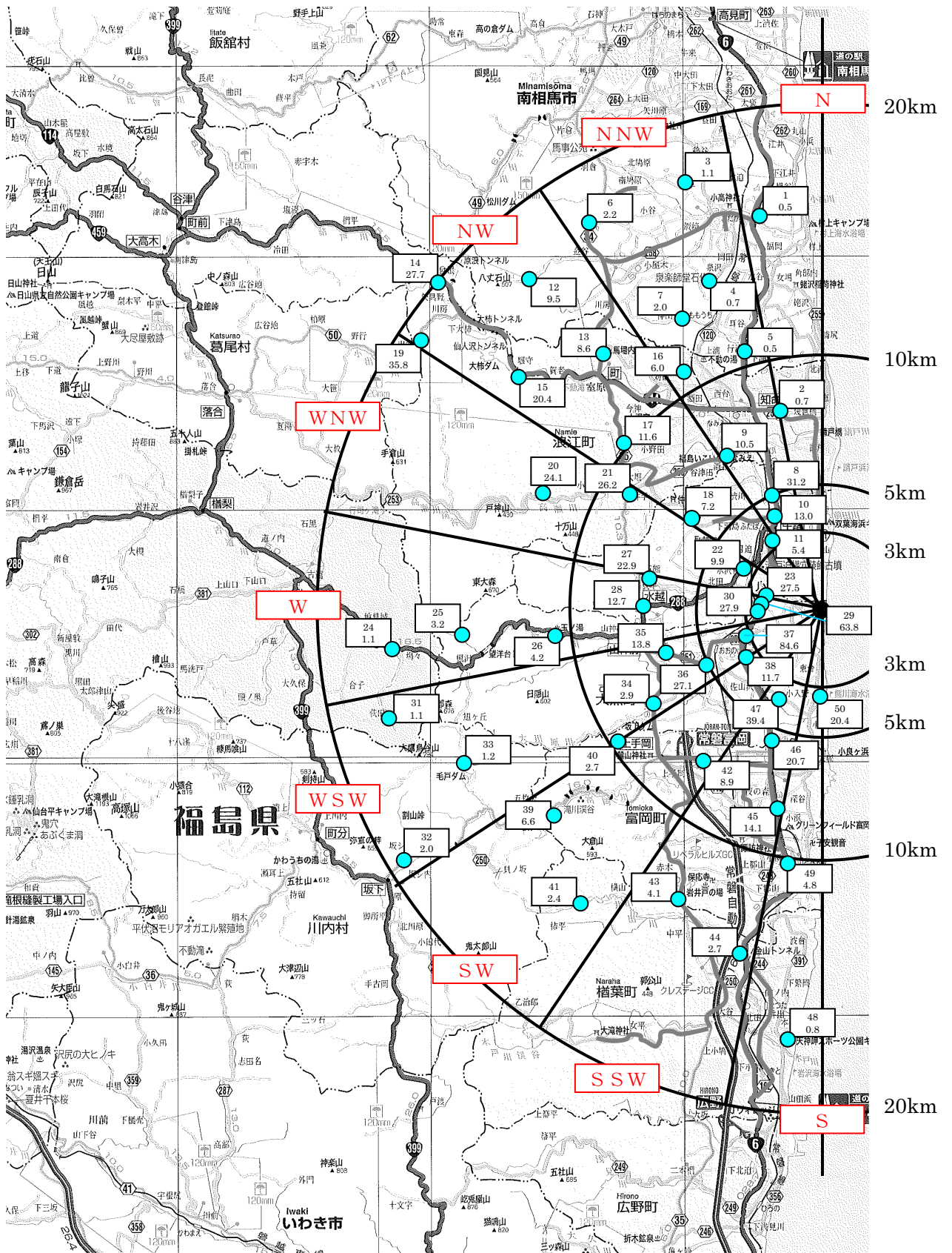
후쿠시마 제 1 원자력발전소에서 20km 권내의 공간 방사선량을 측정 결과 (측정일 : 2011년 5월 13일)
