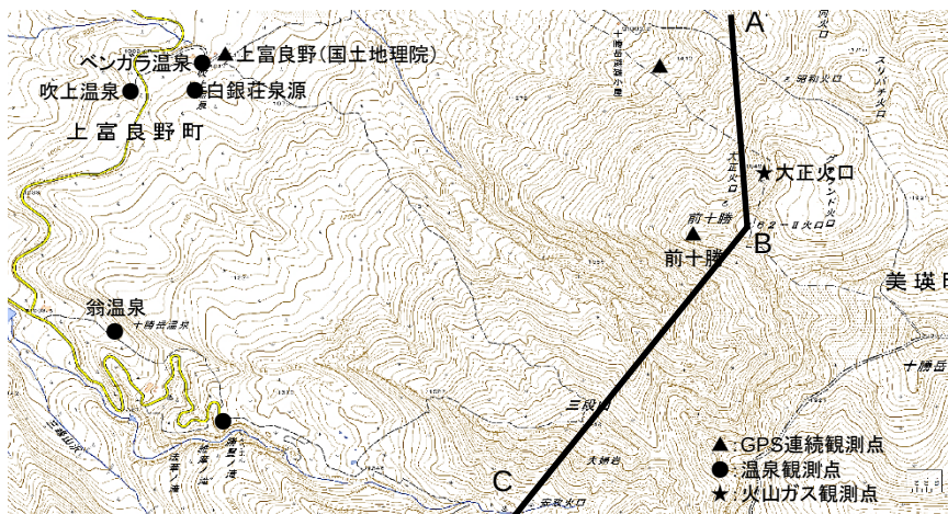
図1 十勝岳における観測点分布
