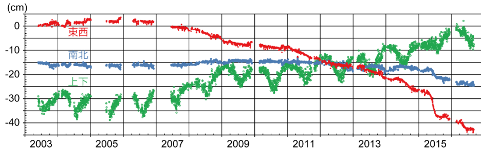
図2 上富良野点(国土地理院)を基準とした前十勝点の変位
