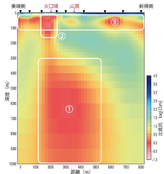
図4 十勝岳を横断する北西-南東測線でのMT探査結果(2次元解析断面図)
