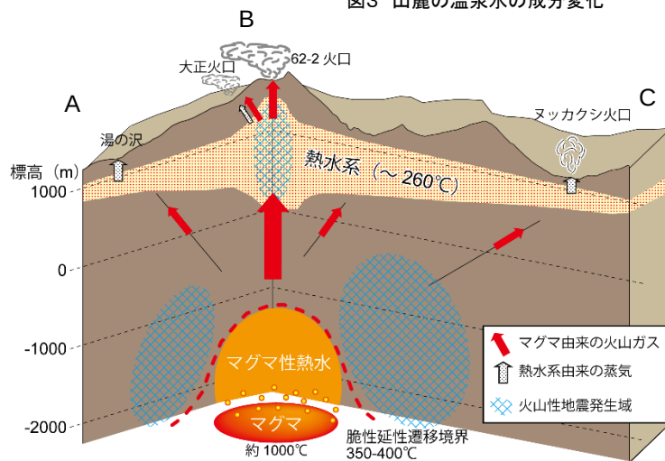
図5 十勝岳の火山体内部構造のモデル図
