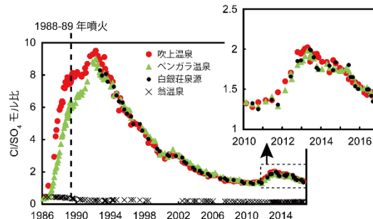
図3 山麓の温泉水の成分変化
