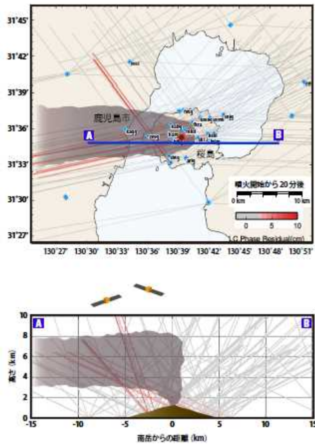
図 13 2012 年 7 月 24 日に桜島南岳において発生した爆発によって放出された火山灰の影響で、GNSS 衛星からの電波に遅延が生じた伝搬経路
