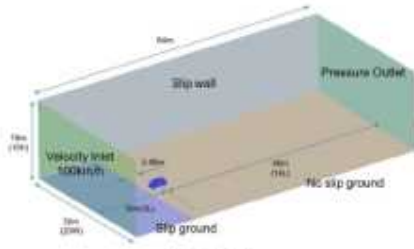
図2. 境界条件
