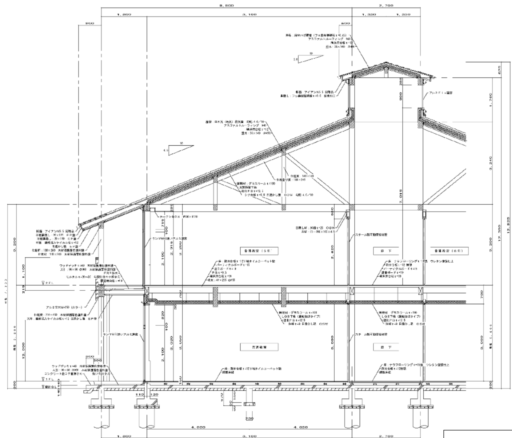
断面詳細図 (Non Scale)
