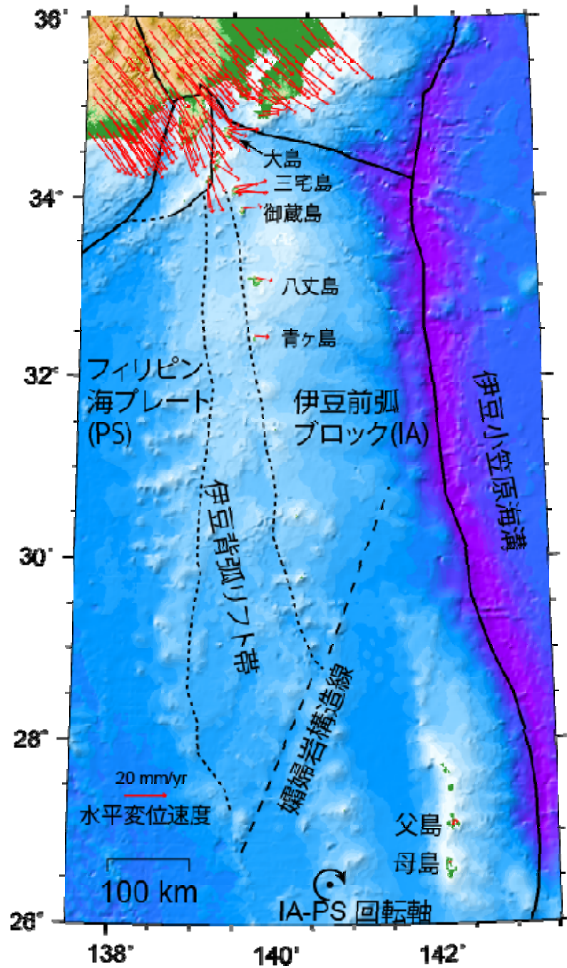
図2. GEONETによる伊豆小笠原諸島の水平速度ベクトル(国土地理院[課題番号:6013])。フィリピン海プレートの剛体部分を基準とした2007年1月から2009年7月までの水平速度ベクトルを示す。伊豆諸島の速度ベクトルが系統的に東向きを示し、背弧拡大に伴う運動を表している。
