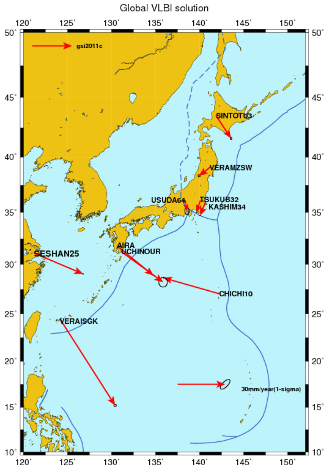
図1．VLBI 観測によって得られた日本列島及び周辺域のプレート運動（国土地理院 [課題番号：6013]）。
