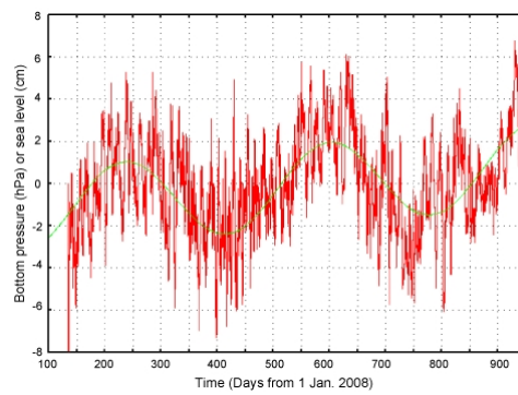
図 3 宮城県沖の海底圧力変動の共通成分の年収変化と経年変化
