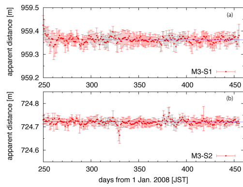
図 2 熊野灘分岐断層で得られた基線長の時系列データ
