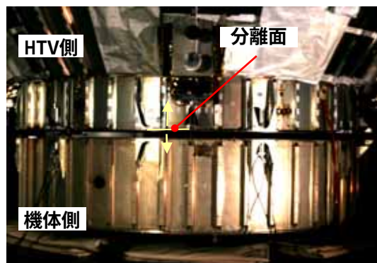
HTV分離部分離試験 (分離直後の写真)
