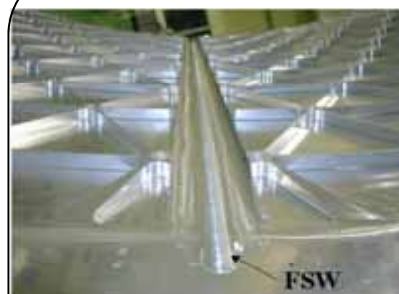
摩擦攪拌接合 (FSW) 概要
