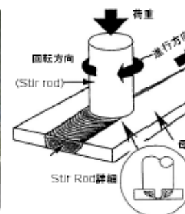
摩擦攪拌接合 (FSW) 概要
