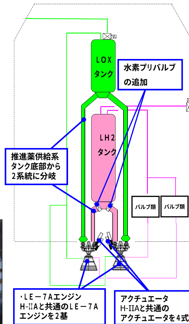
1段推進系 概略
