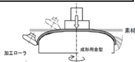
タンクドーム スピニング成形 概要
