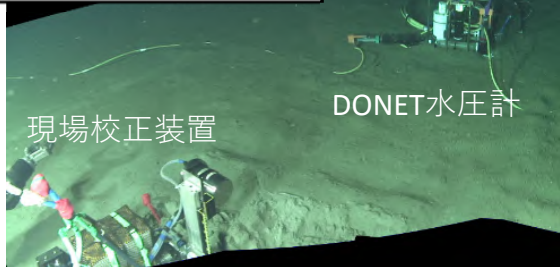
DONETの海底津波計(水圧計)の現場校正
