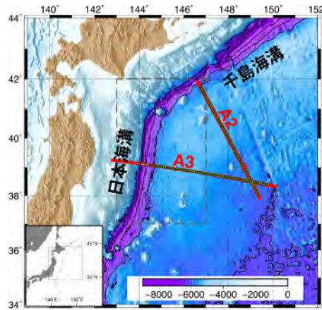
千島海溝付近の海底地形
