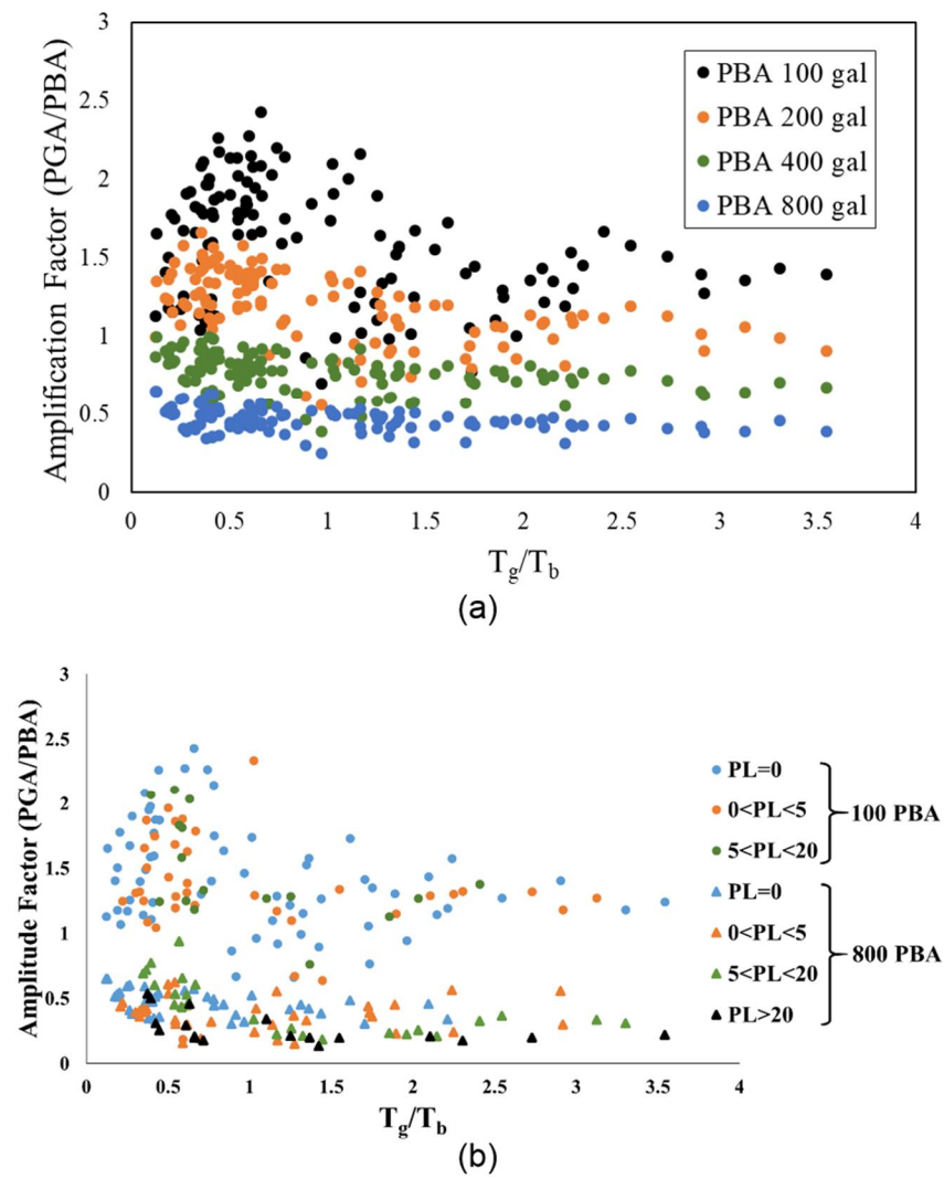
図 3. 逐次非線形解析により得られた表層地盤増幅率 (a) 非液状化解析, (b) 液状化解析 (拠点間連携研究 [課題番号: 2990] )
