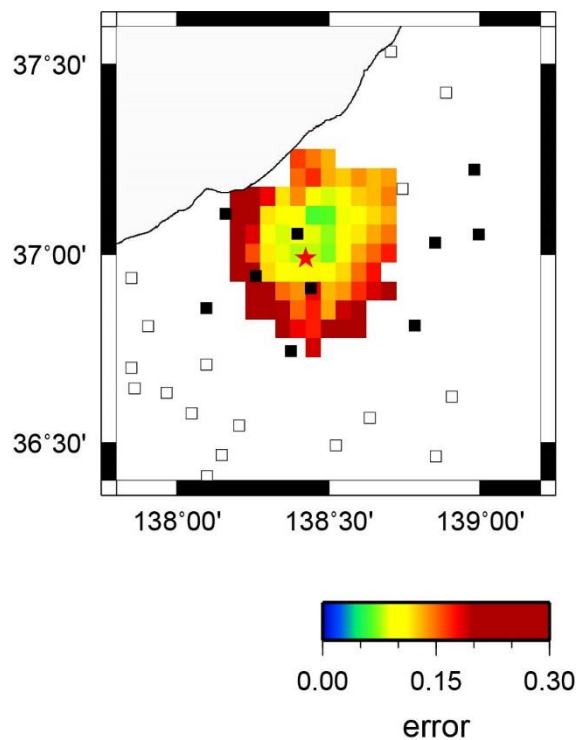
図 8. 観測点間振幅比の再現誤差の分布（赤色星印が土石流発生日点，黒色四角が解析に用いた観測点を表す）（拠点間連携研究〔課題番号：2994〕）
