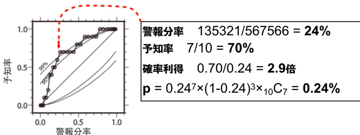
図18. 地震活動静穏化にもとづく予測マップの性能評価（東北大学〔課題番号：1206〕，東海大学〔課題番号：2501〕）
