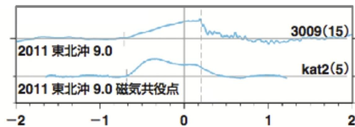
図20. 東北地方太平洋沖地震前後の地磁気共役点近傍のTEC変動(日置, 2018) (東海大学 [課題番号: 2501])
