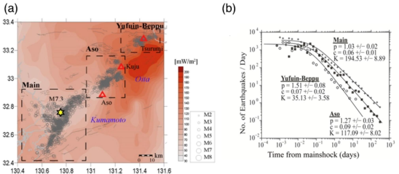
図7. 2016年熊本地震の3つの余震活動域と地殻熱流量, 余震減衰p値との関係(Opris et al., 2018) (東北大学 [課題番号: 1206])
