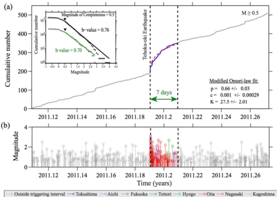
図6. 遠地誘発地震活動がみられた地点での東北地方太平洋沖地震前後の地震活動の時系列(Opris et al., 2018) (東北大学 [課題番号: 1206]) (a) すべての地点をスタックした地震活動積算曲線。東北沖地震後の7日間の活動は青線で示す。赤破線は大森-宇津則による理論曲線。左上は前期間のM-頻度分布。(b) 同じ期間のMTダイアグラム。東北沖地震後のステムプロットの色は地域毎に変えている。
