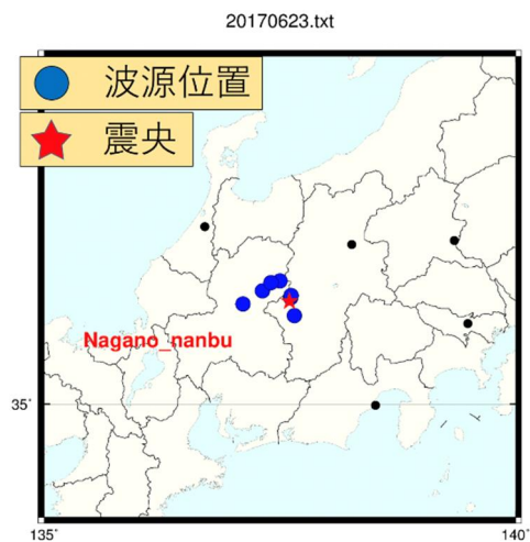
図22. 長野県南部の地震 (M5.6, 深さ7km) の震源付近から2日前に放射されたVLF帯パルス電磁波 (東海大学 [課題番号: 2501])
