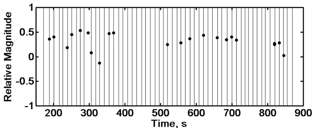
図17. 図16の実験で見いだされた最大のクラスターを構成するリピーターの前震の発生時刻と相対マグニチュードの関係（立命館大学〔課題番号：2402〕）
