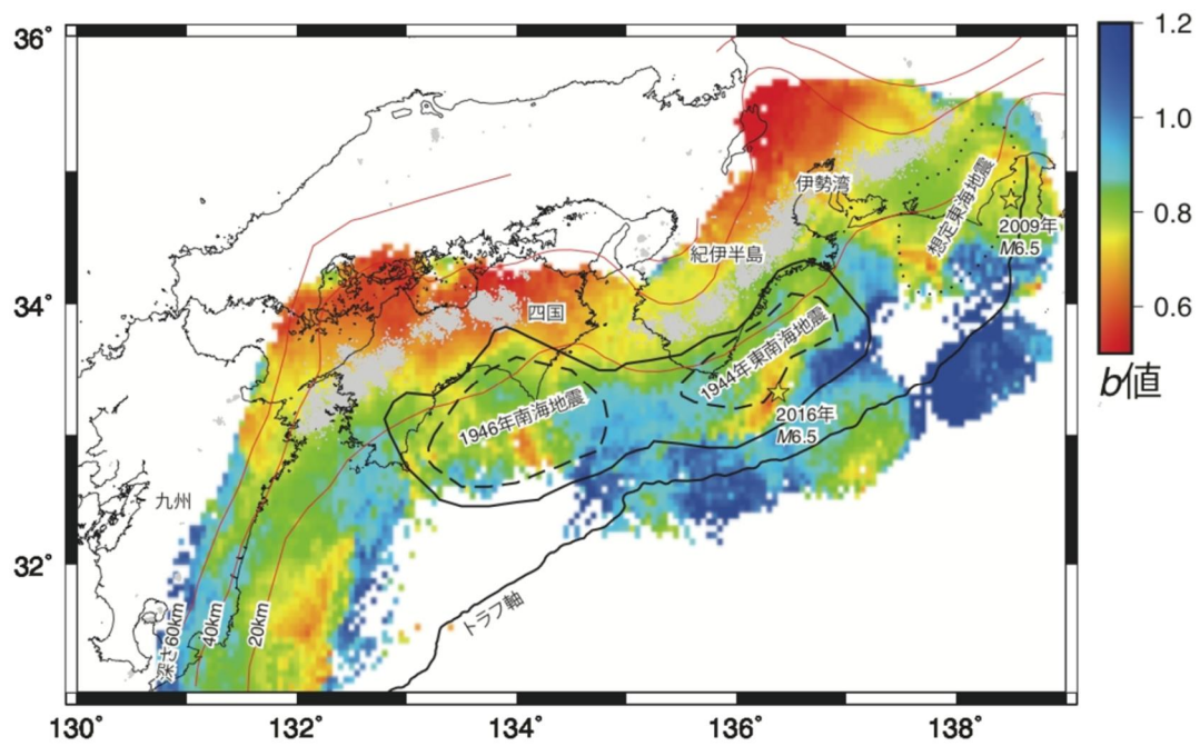
図10. 南海トラフ沿いのb値分布(楠城・吉田, 2017) (東京大学地震研究所 [課題番号 : 2902] )
