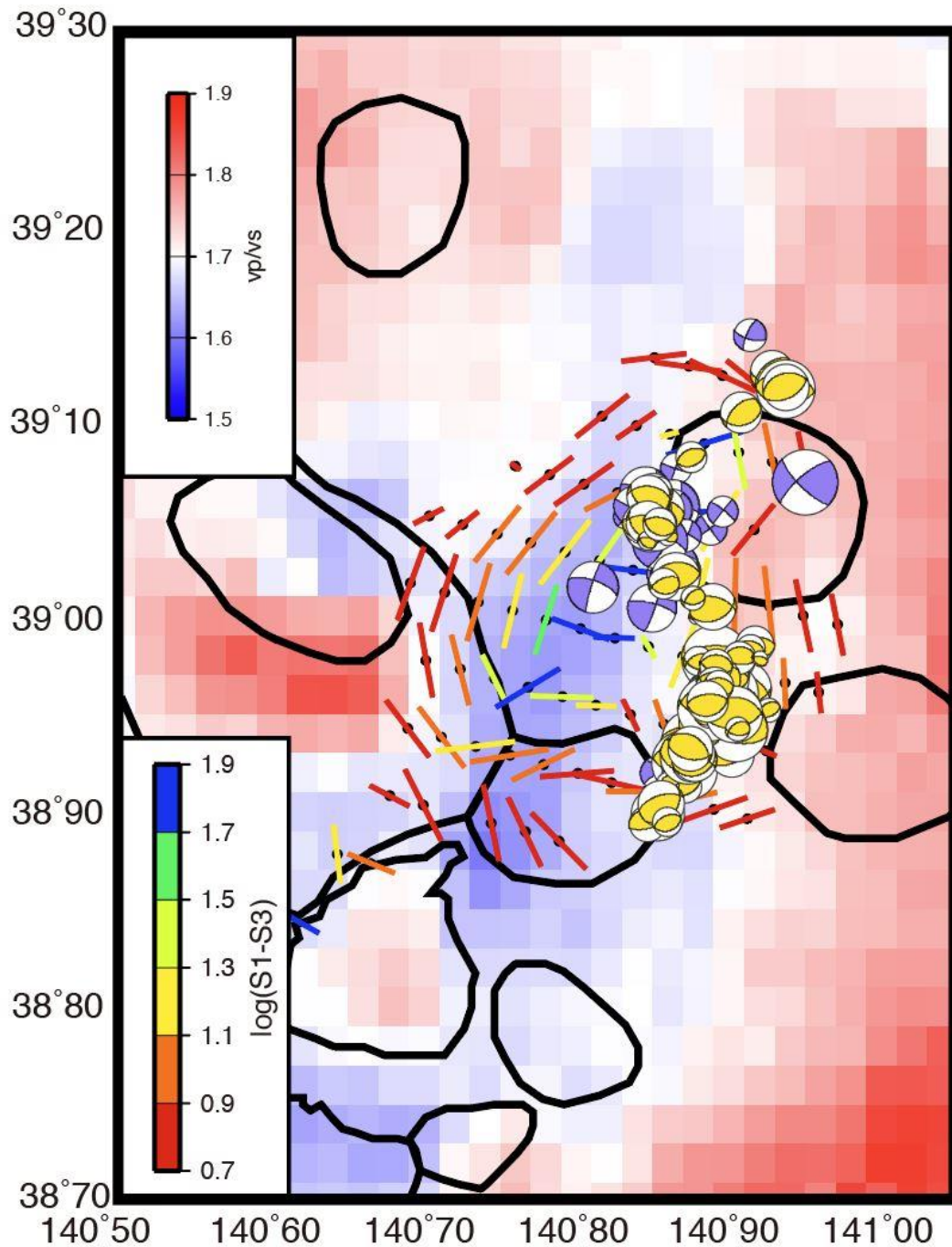
図 5. 2008 年岩手・宮城内陸地震の特異な余震と応力場と V_p/V_s 比構造の比較。
