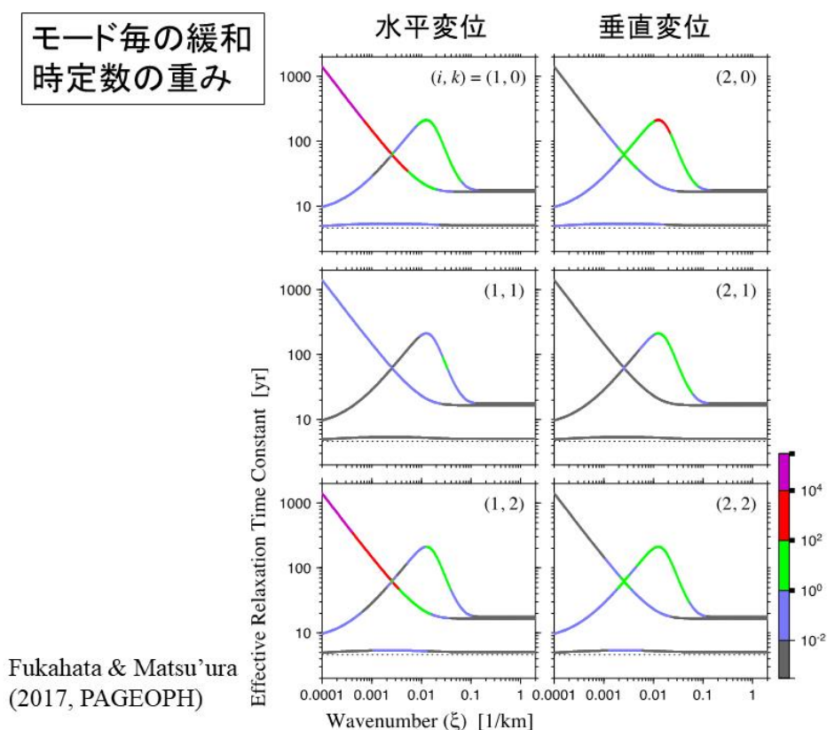
図 6. 各緩和時定数の重みは、係数 a_{ikm} で表される。この図は、その係数の大きさの空間波数依存性を示している。係数の大きさが桁で変わること（右下のカラーバーがスケール）。紫や赤の部分が、粘性緩和において主要な役割を果たす。つまり、非常に長波長（数百 km 以上）の水平変位については、 \tau = 4.6 年にも拘わらず、実際の緩和には数百年以上もの時間がかかることが分かる（左上・左下図）。垂直変位についても、50 ~ 100 km の波長の変形が、100 年以上の緩和時間を持つことが分かる（右上図）。実際の緩和には名目的な Maxwell 緩和時間 \tau よりもずっと長く時間がかかることの原因である。ただし、なぜ緩和時定数が 3 つあるのか、またなぜそれらに波数依存性があるのかという問題については、数学的には非常に明らかであるが、物理的に説明することはなかなか難しい。（京大防災研[課題番号：1905]）。
