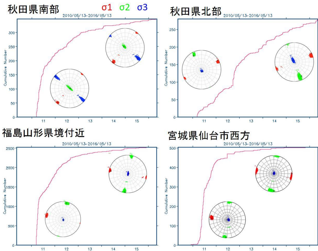
図 3. 東北沖地震後に活発化した内陸群発震源域での応力場。
