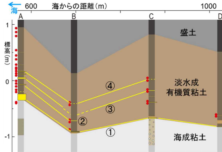
web公開の元となる高知県南国市の地質柱状図①~④の4層の堆積物が内陸奥まで確認できる。(Tanigawa et al., in pressに基づく)
