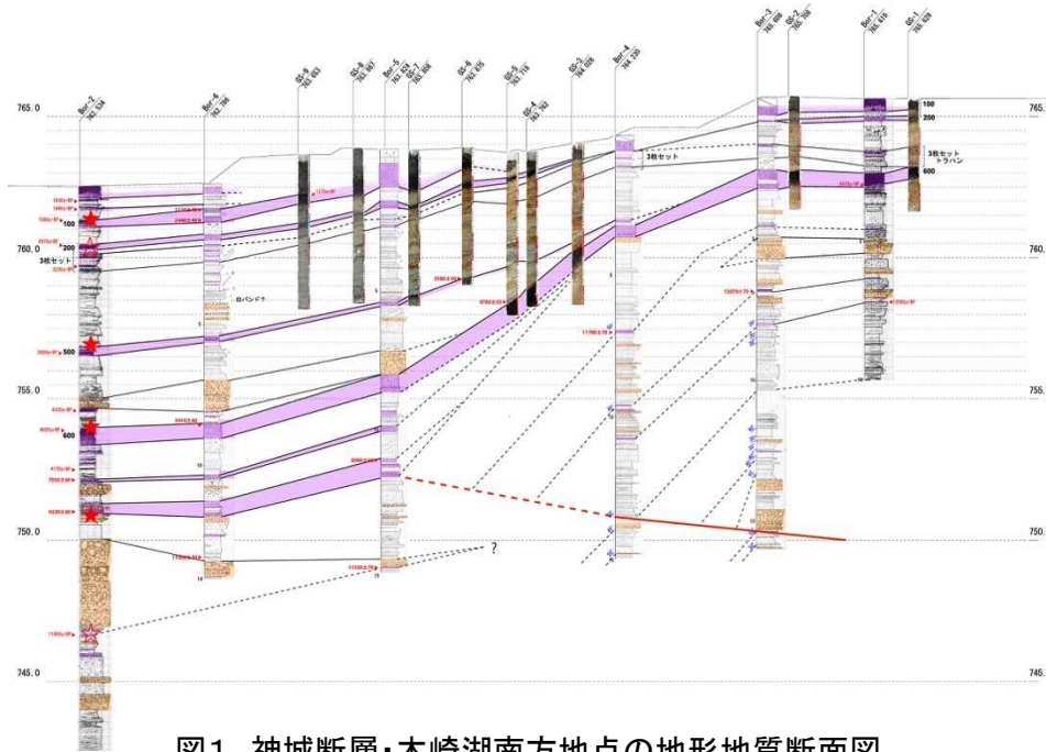
図1 神城断層・木崎湖南方地点の地形地質断面図
