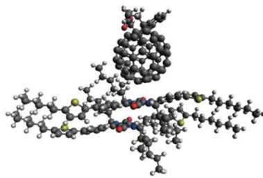
太陽電池の全系シミュレーション
