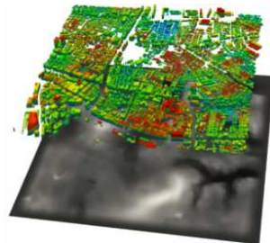
津波の遡上予測
