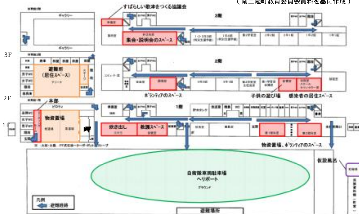
図表 2-1-12 歌津中学校、伊里前小学校配置図 (南三陸町教育委員会資料を基に作成)
