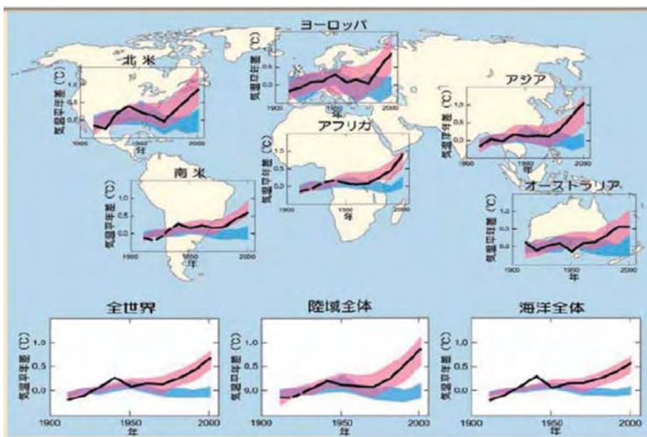
世界規模及び大陸規模の気温変化
