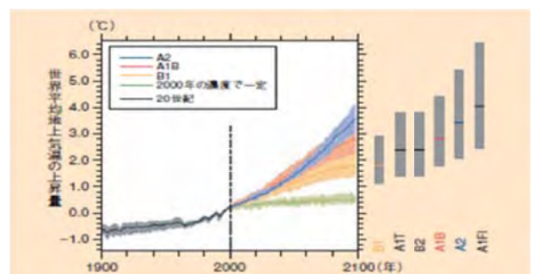
今後の気温上昇の予測
