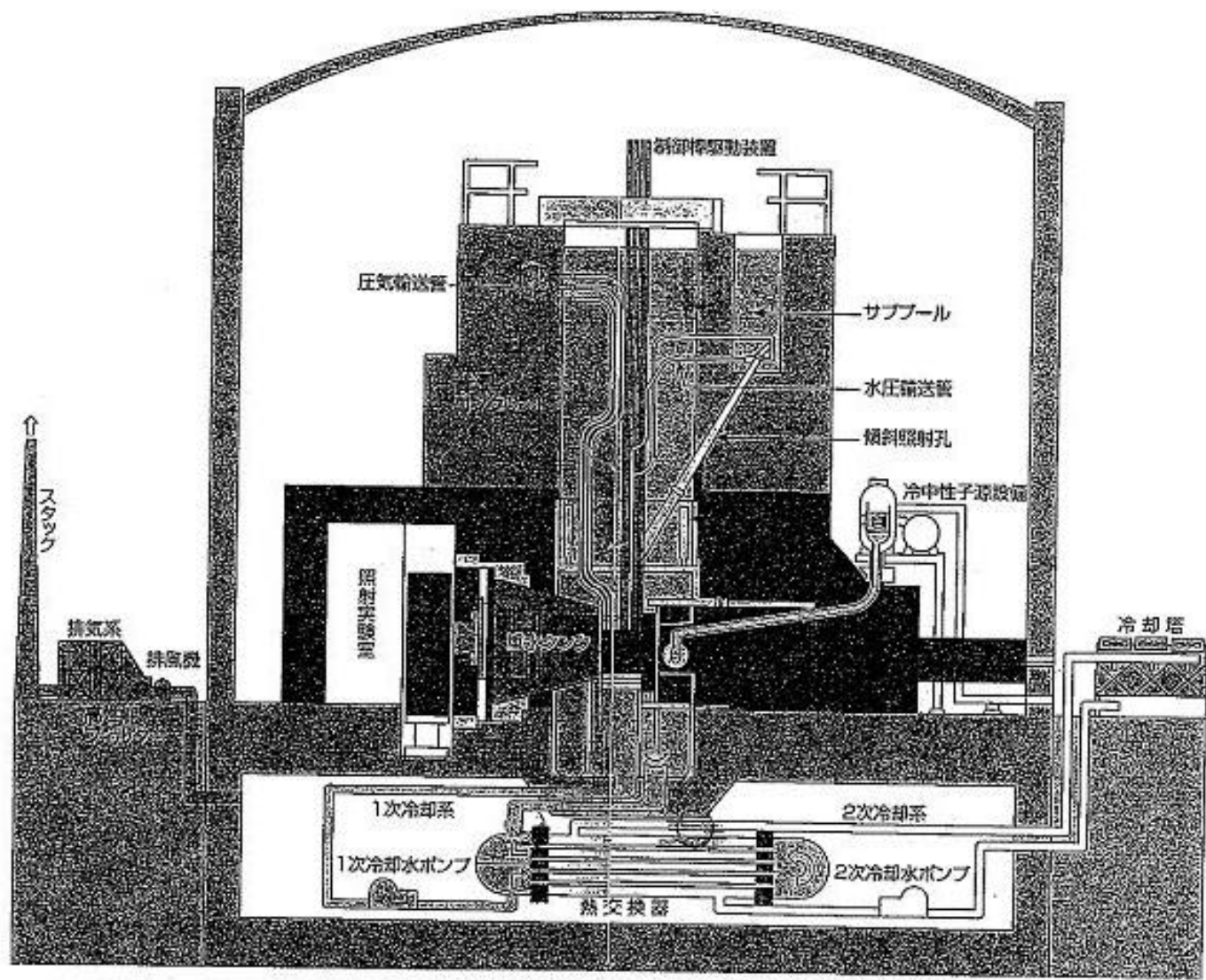
京都大学 KUR 冷却系統概略図
