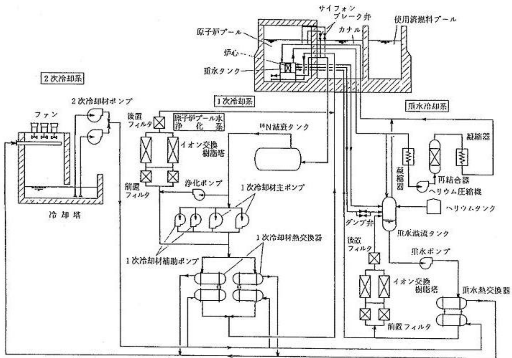
日本原子力研究所 JRR-3 冷却系統概略図
