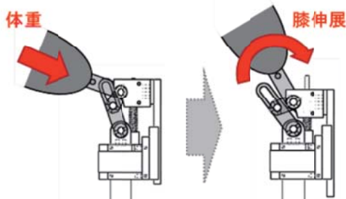
階段昇段できる高機能大腿義足(機構図)
