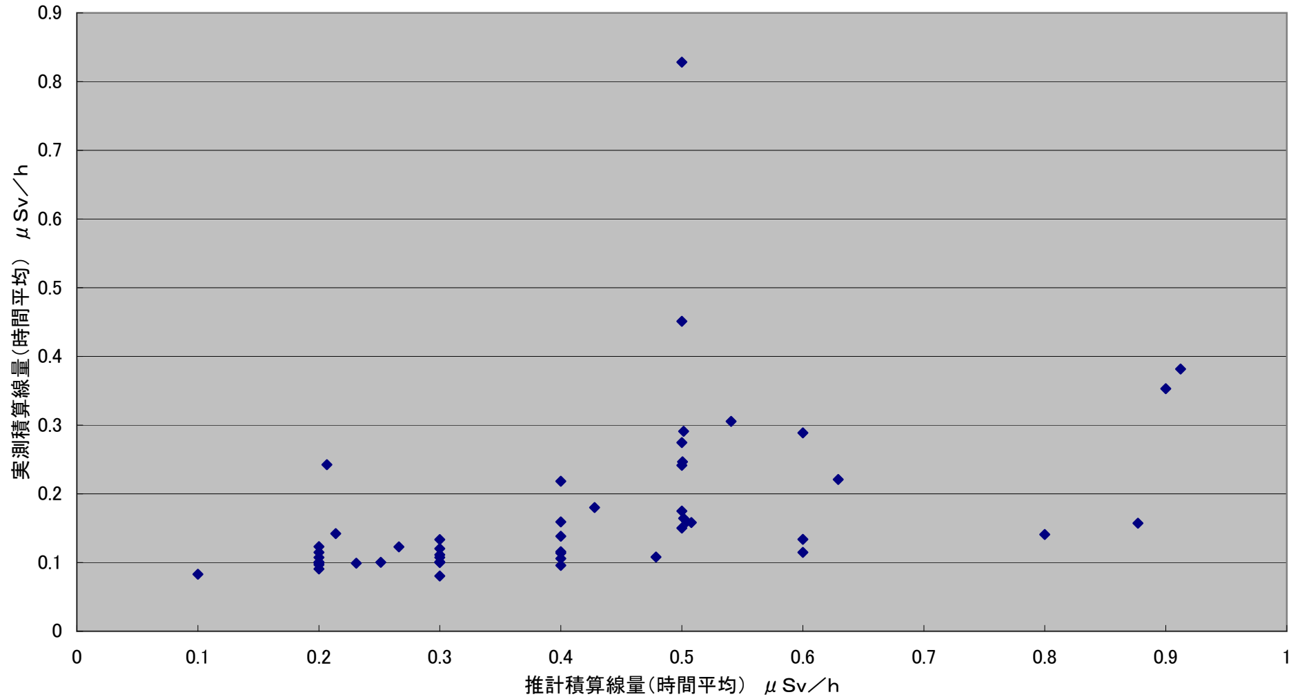
推計積算線量(時間平均:校舎内窓際)と実測積算線量(時間平均)の比較 (平成23年5月23日~6月5日)
