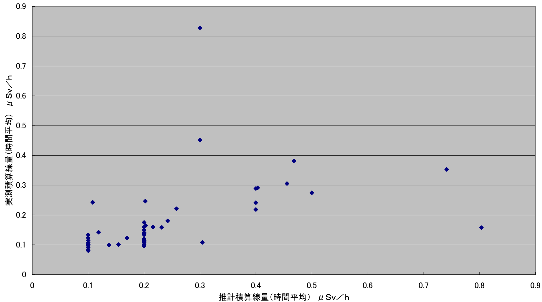
推計積算線量(時間平均:校舎内中心)と実測積算線量(時間平均)の比較(平成23年5月23日～6月5日)
