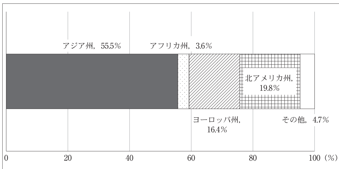
グラフ 2 州別の二酸化炭素排出量の割合 (2015 年)
