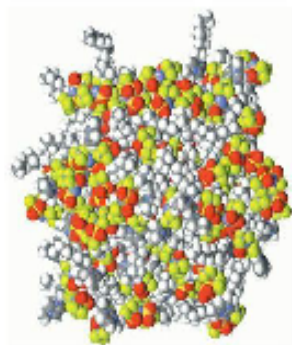
分子動力学法で計算したイオン液体の構造
