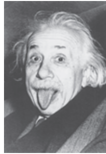
アインシュタイン
