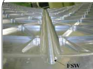
摩擦攪拌接合 (FSW) 概要
