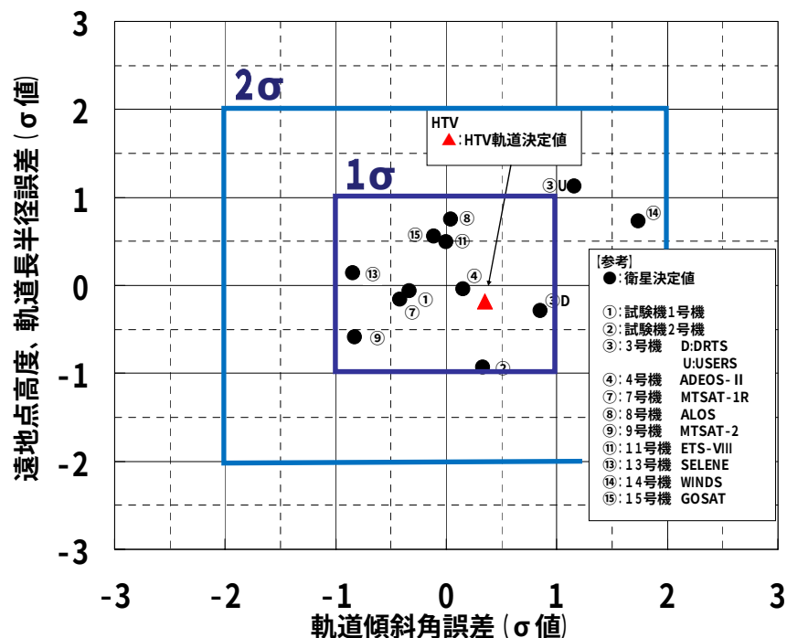
軌道投入精度
