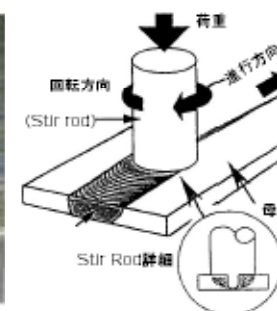
摩擦攪拌接合 (FSW) 概要
