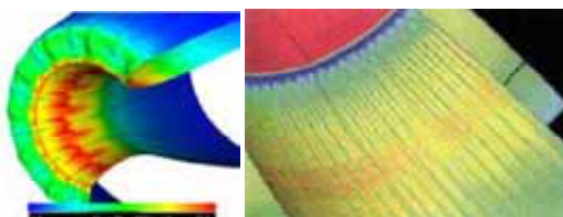
エロージョン解析の高度化
