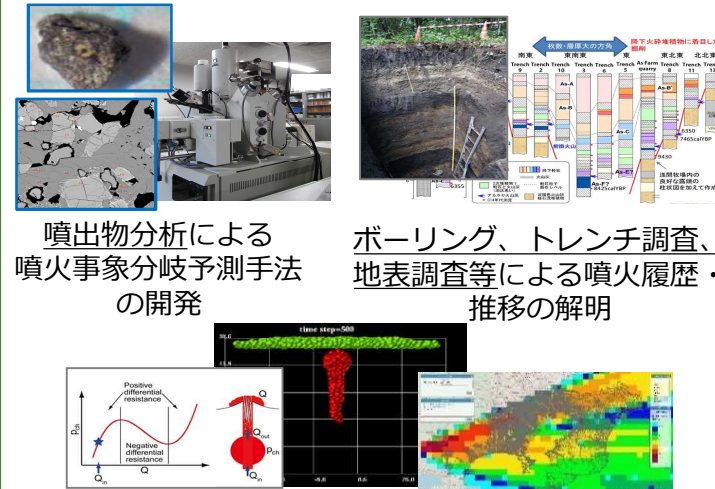
数値シミュレーションによる噴火ハザード予測（マグマ移動、噴火ハザードシミュレーション）
