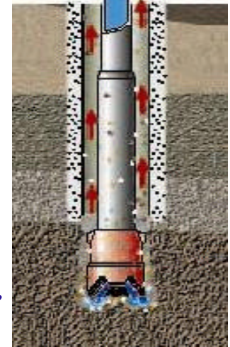
泥水循環
