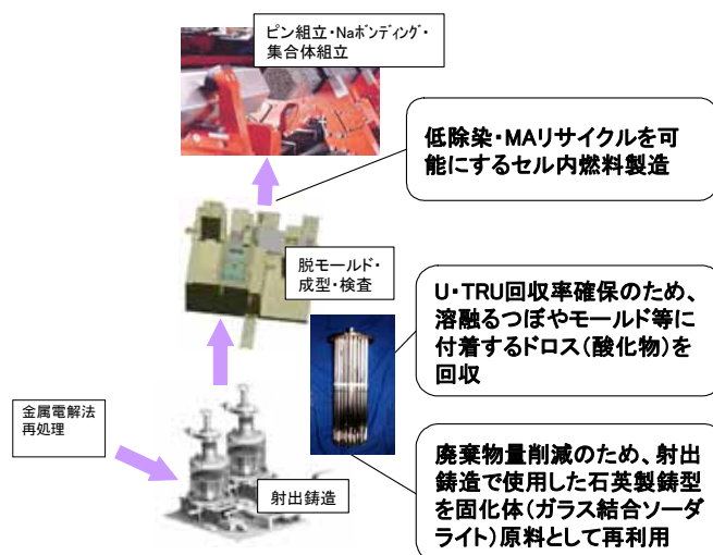
図1-1-14 射出鑄造法燃料製造の概念図
