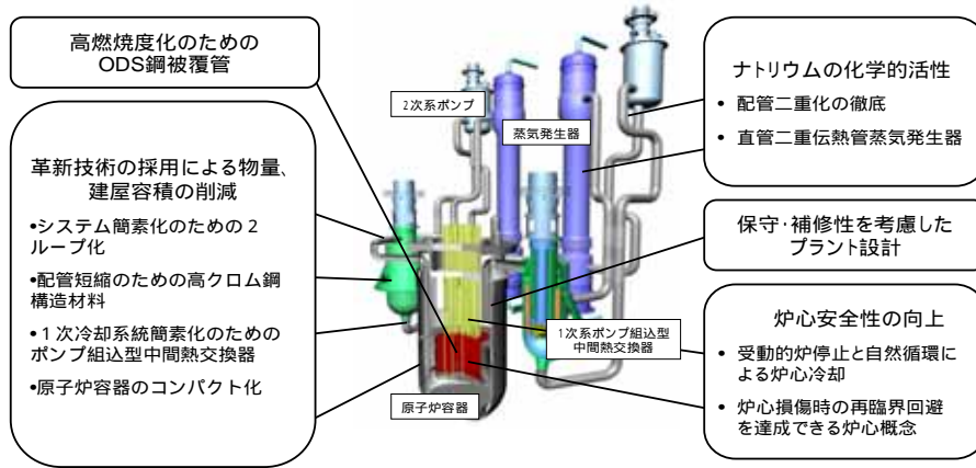
図1-1-4 ナトリウム冷却高速増殖炉概念図
