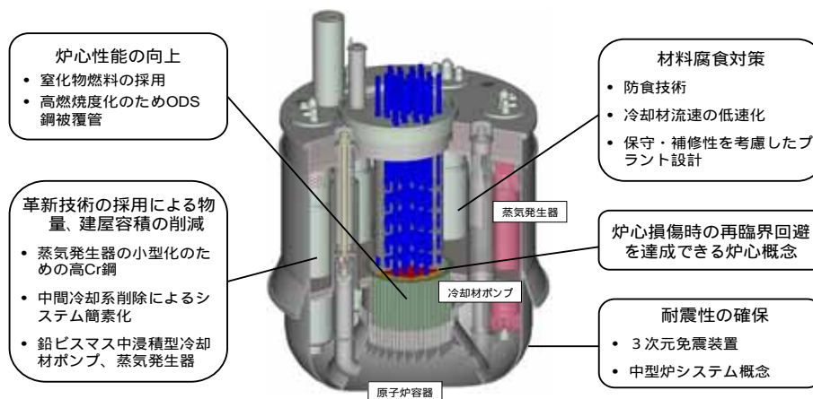
図1-1-6 鉛ビスマス冷却高速増殖炉概念図
