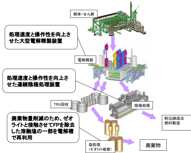
図1-1-10 金属電解法再処理の概念図
