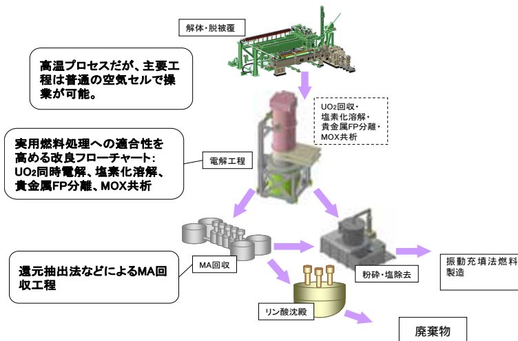
図1-1-9 酸化物電解法再処理の概念図
