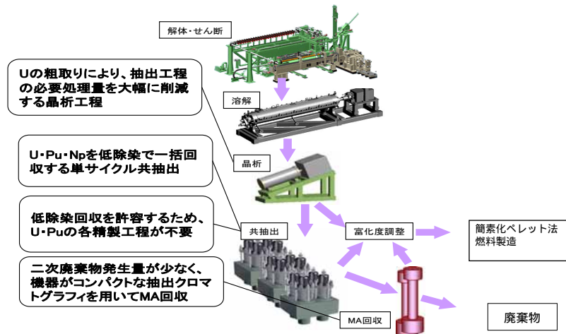
図1-1-8 先進湿式法再処理の概念図
