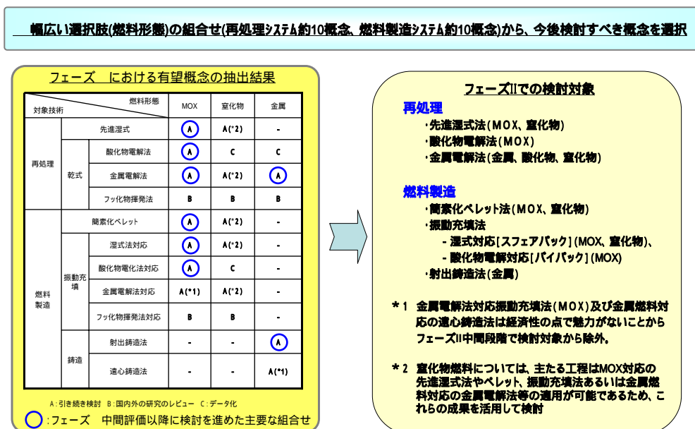
図1-1-2 実用化戦略調査研究の実施方針 フェーズIIでの検討対象：燃料サイクルシステム
