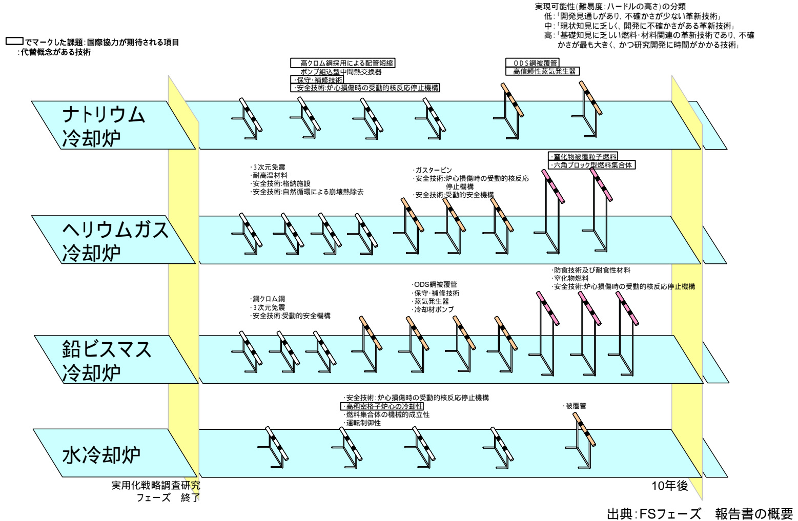
図1 - 1 - 17 各高速増殖炉候補概念の技術的実現性
