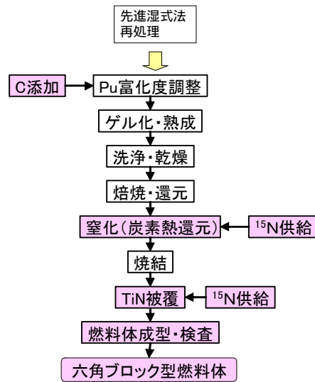
図1-1-15 被覆粒子燃料製造の概念図
