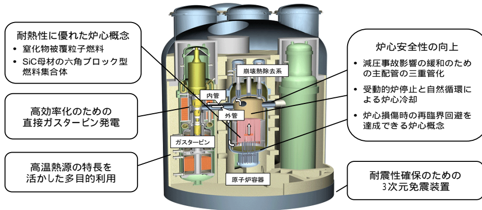
図1-1-5 ヘリウムガス冷却高速増殖炉概念図
