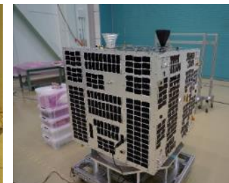
残留磁気測定試験
