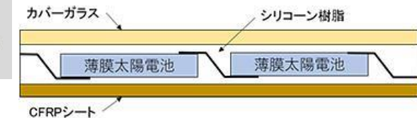
今回のパネル構造
