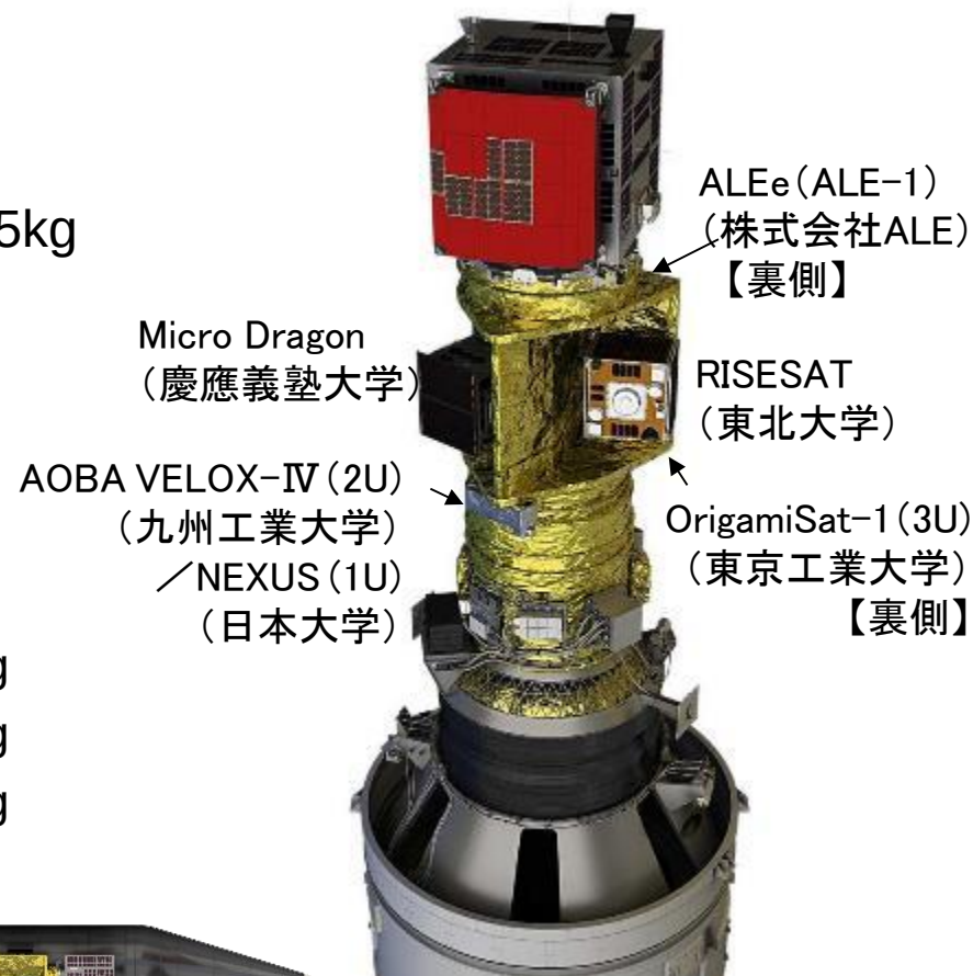
小型実証衛星1号機 (RAPIS-1)
