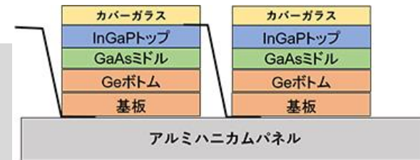
今回のパネル構造
