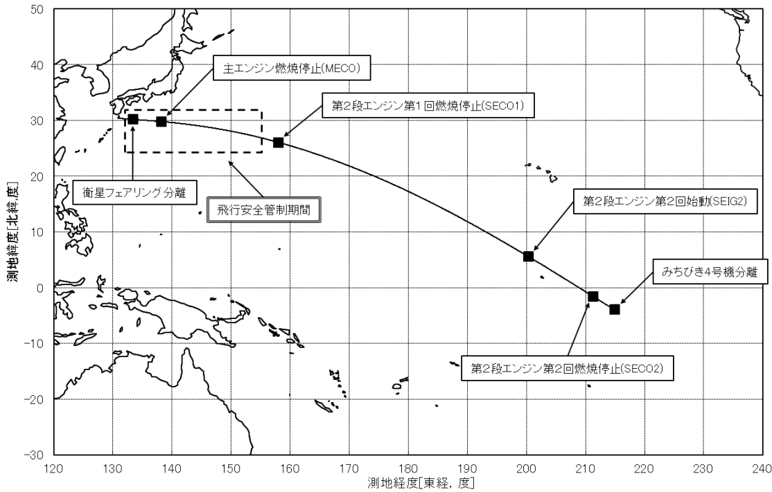
H-IIA・F36 シーケンス・オブ・イベント
