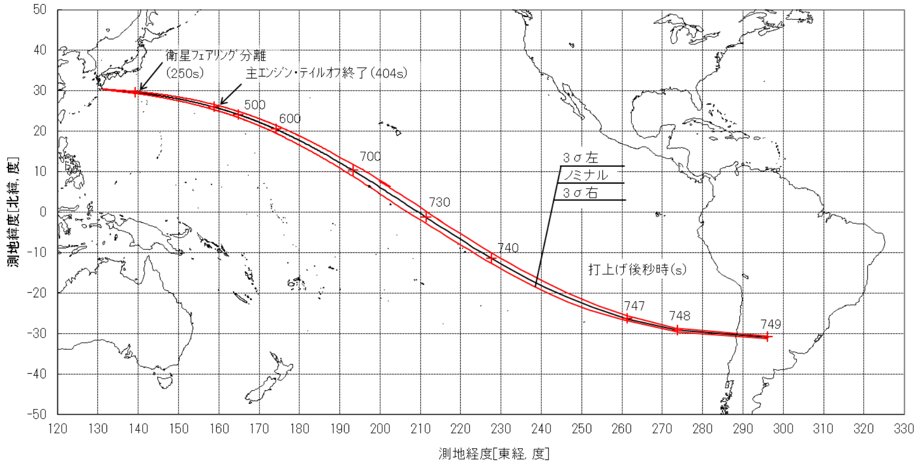
図10: ロケットの落下予測点 (注) 軌跡と3 \sigma 分散範囲
