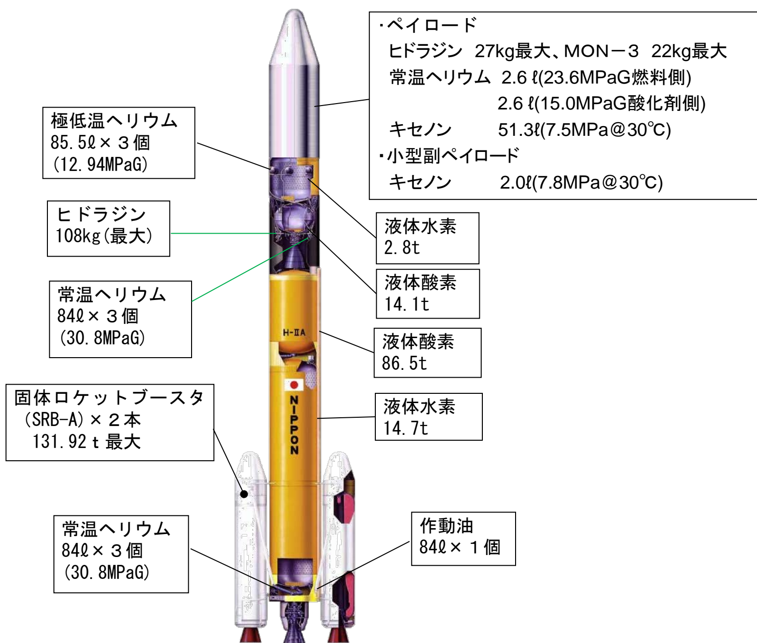
図1: ロケット等搭載用保安物
