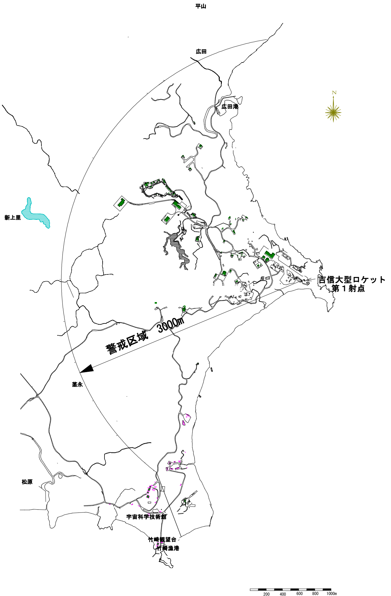
図-2 打上げ時の陸上警戒区域
