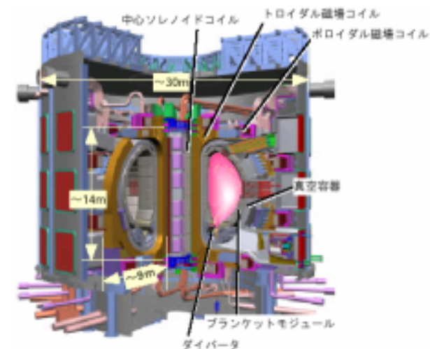
ITER本体概要図
