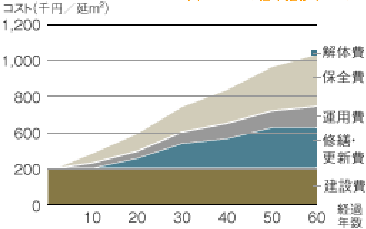
図3: LCCの経年推移イメージ
