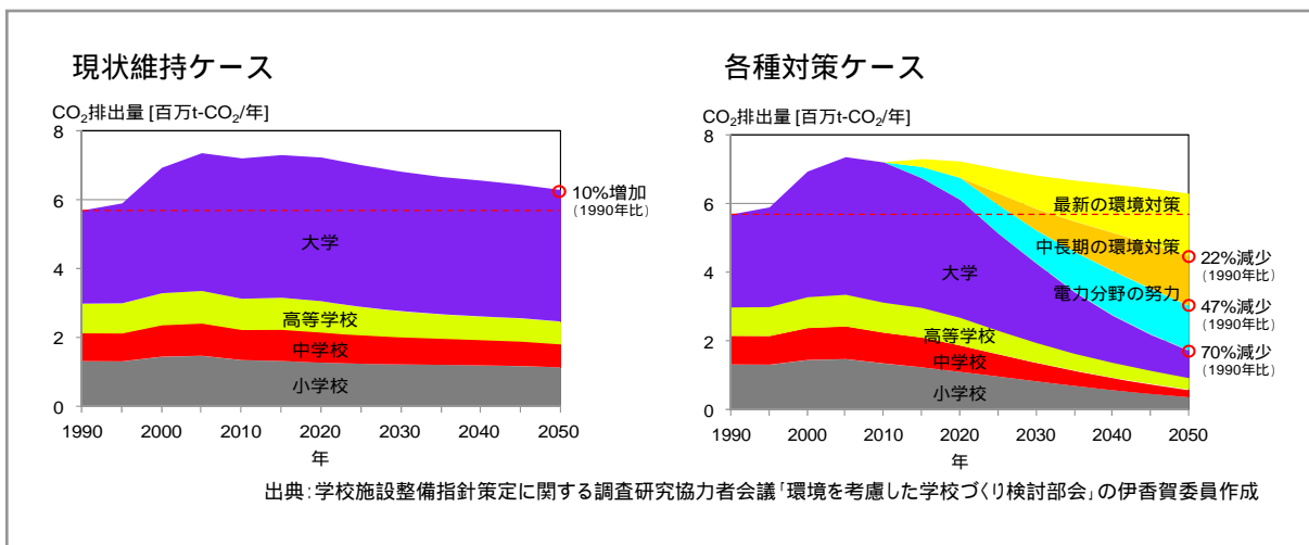
図表16 CO 2 排出総量のマクロ推計
