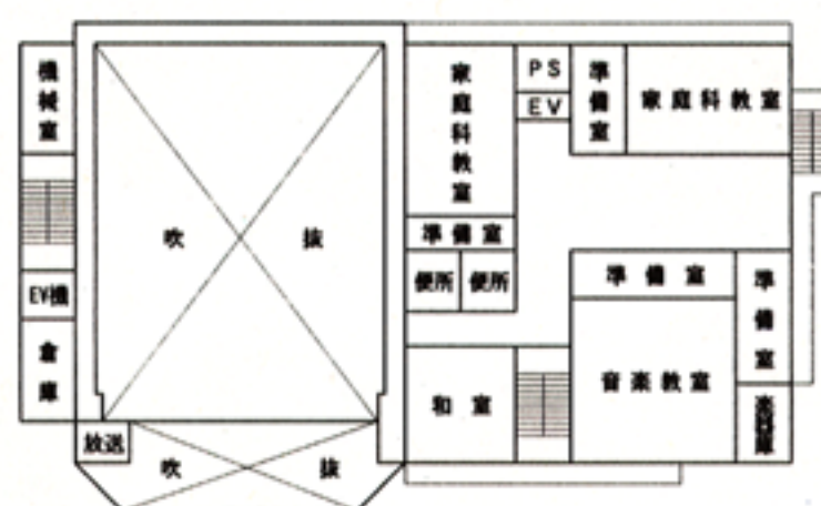
6 階平面図
