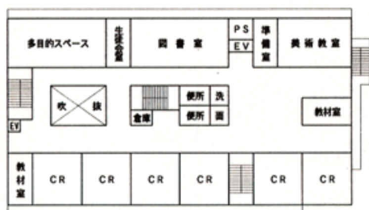
3 階平面図
