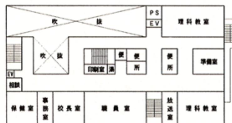
2 階平面図
