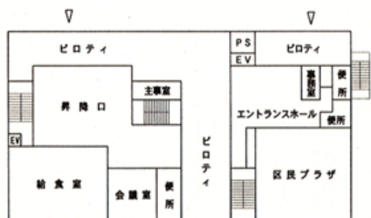
1 階平面図
