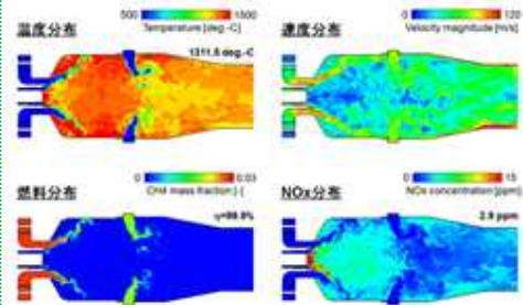
L30A-DLE燃焼器中心断面における各物理量分布
