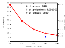
RSDFT-CPMD法1ステップの計算時間および実行効率のCPU数依存性(赤:初期の実装、青:最終的な実装での結果)
