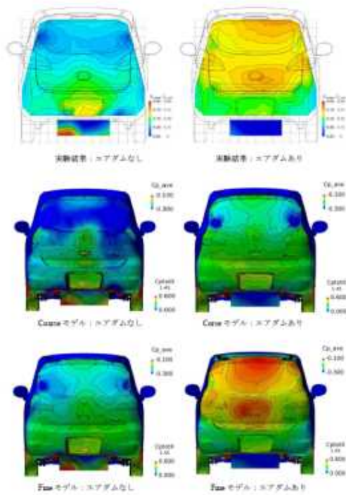
図6. バックドア圧力分布(実験-Cp=0.05~0.25, 計算-Cp=0.1~0.3)
