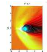
「京」を用いた高解像度計算結果で得られた弱磁化小天体近傍のイオン密度及び磁力線のプロファイル
