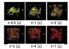
乱流中における雲粒子の成長と分散の時間発展
