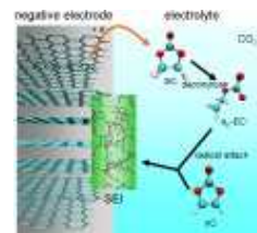
リチウムイオン電池内におけるVC添加剤とEC電解液の反応
