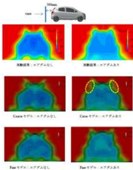
図4. 車体後方 300km Total pressure(0.5~1.0)
