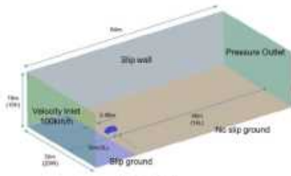
図2. 境界条件
