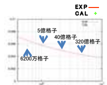
全抵抗係数 (試験と計算の比較)
