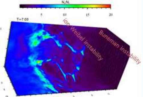
高マッハ数衝撃波の3次元構造 (色は電子密度を表す)
