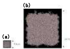
分子構造計算結果 (a) 先行研究, (b) 本研究
