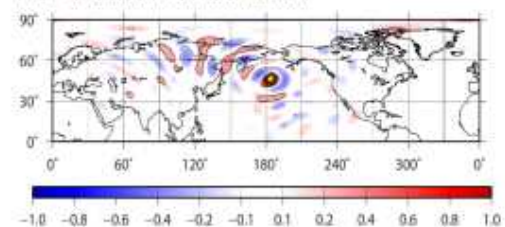
アサンブルデータ同化による18日目の水蒸気量の 相関マップ(理化学研究所プレスリリースより)
