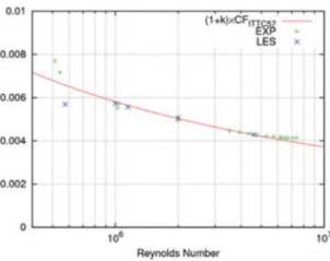
推進抵抗の比較 提供: 一般財団法人
