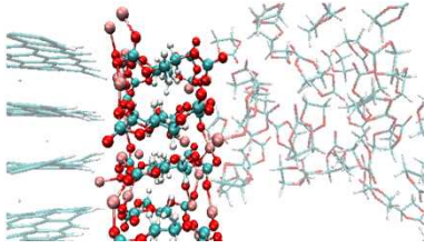
図1:Liイオン二次電池負極界面における界面保護膜(中央部)形成のシミュレーション。左側は炭素電極、右側は電解液。
