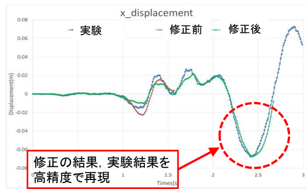
E-ディフェンス実験で計測された構造物の地震応答の再現
