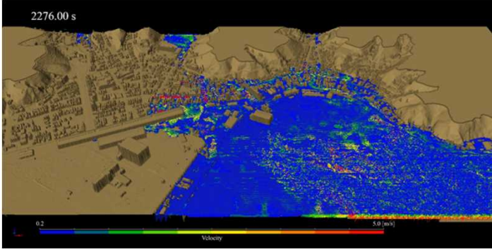
2011年東北地方太平洋沖地震による津波の釜石市の再現計算(高解像度3D計算により津波波力を高精度に評価する)
