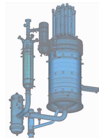
高温工学試験研究炉 の時刻歴応答解析結果
