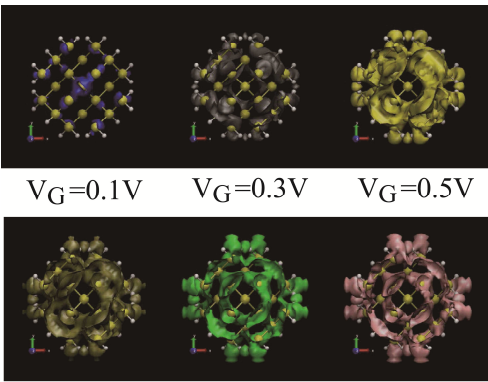
図1 SiナノワイヤFETでのチャネルを流れる電流密度のチャネル断面での分布。ゲート電圧変化により、界面の影響が異なる。
