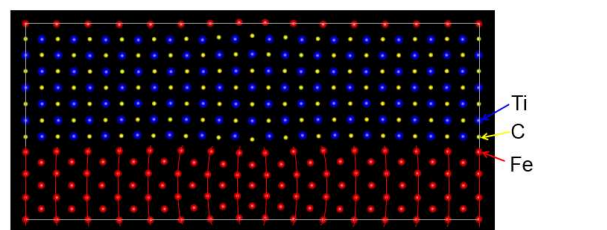
図1 Fe/TiC部分整合界面の安定原子配列 整合界面(赤)と部分整合界面(青)の比較による臨界サイズの決定。横軸: 粒子サイズ、縦軸: 界面エネルギー+歪エネルギー
