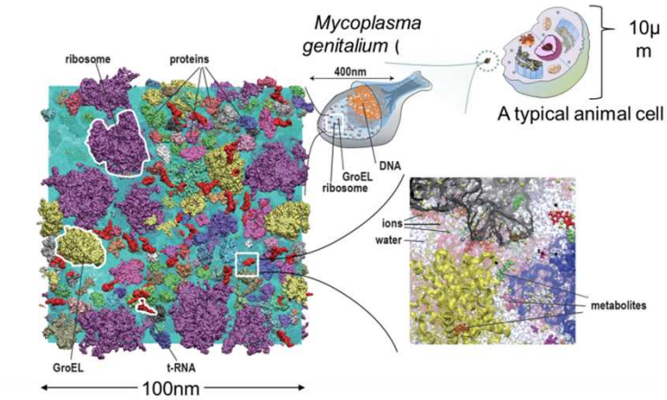
バクテリア細胞質の約10%を表現する全原子モデルに基づく分子動力学計算を実施
