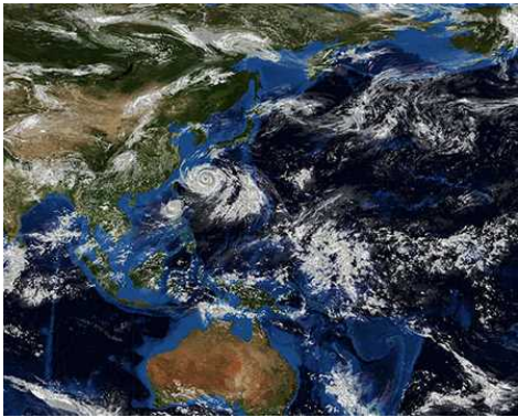
全球雲解像モデルで 計算された雲と台風
