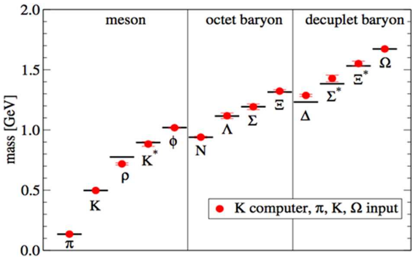
① 京を用いたハドロン質量の計算値(赤)が実験値(黒)を完全に再現
