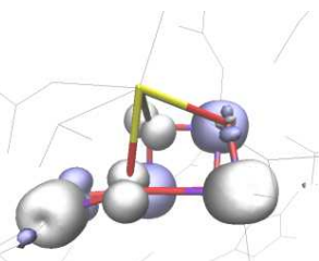
図2: PSIIマンガクラスタ: S 2 基底状態スピン密度
