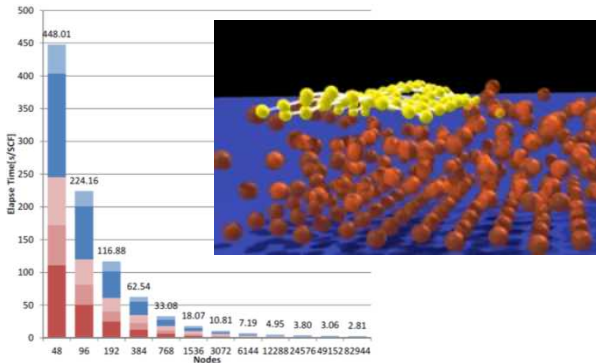
第一原理プログラムPHASE/0は「京」全ノードまでの優れた並列性能を示し、グラフェン成膜プロセスの実温度でのダイナミクス解析により静的計算では獲得できない特性を明確にした。
