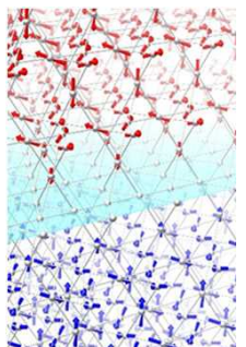
図2: イリジウム酸化物の磁壁。この磁壁に初の金属的可動トポロジカル界面が実現されることを予言し、その後実験で実証された。
