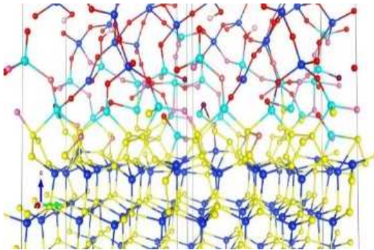
実温度によるダイナミクス解析により、SiC酸化膜界面における従来想定されていなかった欠陥構造をはじめて明らかにし、層状酸化による欠陥低減の可能性を提示した。
