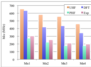
図3: 超微細構造定数(S 2 )
