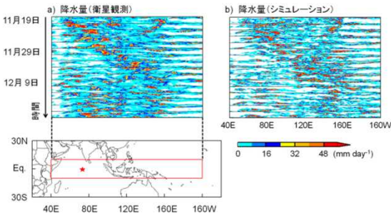
MJO予測の検証例 赤道上の降水量 経度(横軸)ー時間(縦軸)断面図 (左)観測 (右)シミュレーション
