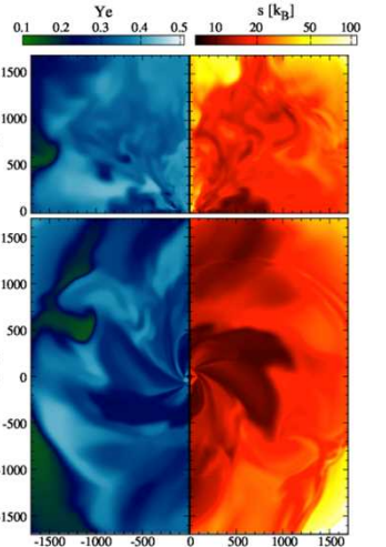
中性子星の合体後に物質が飛び散る様子。左が電子の豊富さを、右がエントロピーをあらわす
