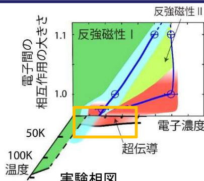
実験相図 図1: 鉄系超伝導体で得られた計算相図(側面)とこれに一致する実験相図(下面)。
