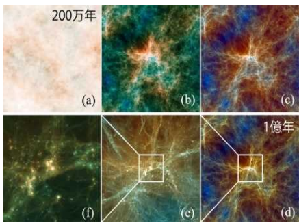
最小質量ハローの形成過程
