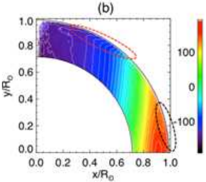
シミュレーションで得られた太陽の回転速度分布。楕円で囲んだ領域で回転速度が急激に変化している。
