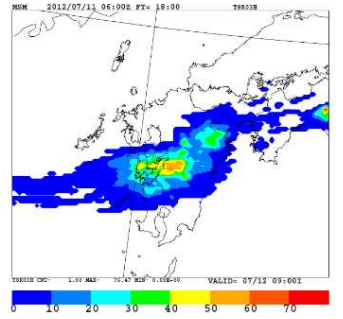
九州北部豪雨についての大雨確率予測分布図
