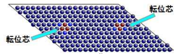
図2 Fe中らせん転位芯計算用スーパーセル Si原子と転位芯の相互作用を転位芯からの距離の関数で示す。Siの場合、強い引力が働くことがわかる。
