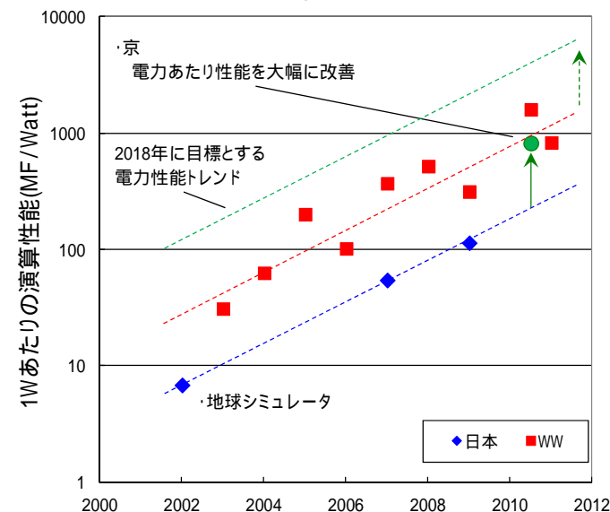
図1. 1Wあたりの演算性能の推移
