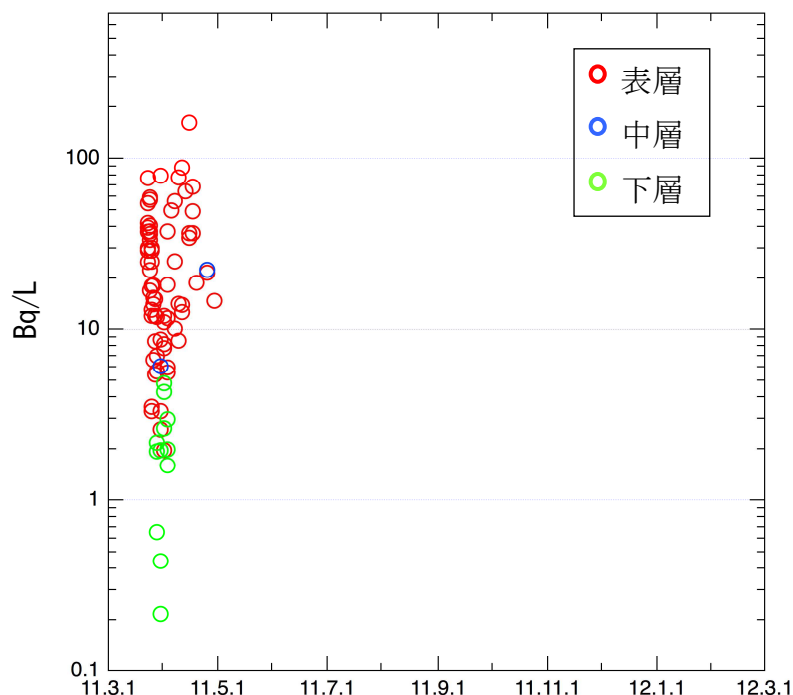
図 II (7) 宮城・福島・茨城県沖における 海水中の ^{131}\text{I} 濃度の時間変化
