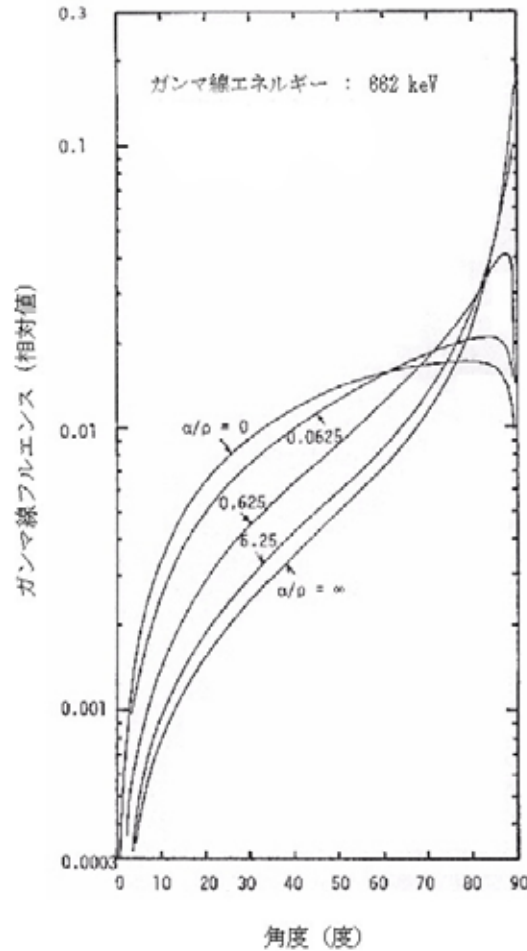
図 4.2 地上高 1m における 線の入射角度依存性
