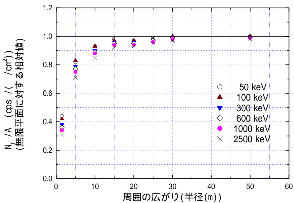
図 D.4 周囲の広がりによる計測値への影響 (検出器 : p 型 : 10g/cm 2 )
