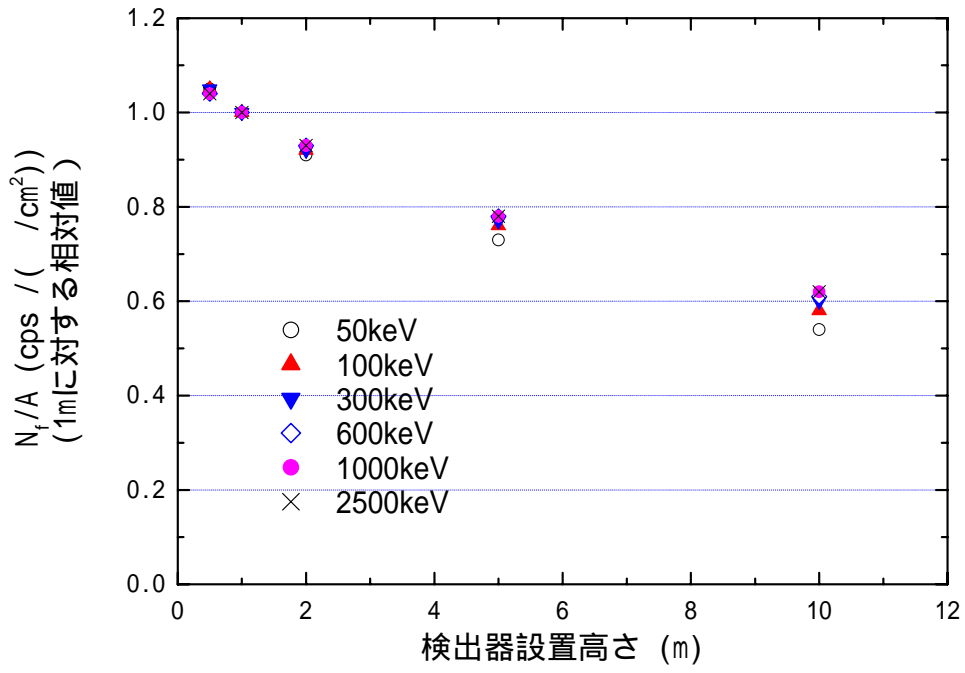
図 D.13 検出器設置高さによる計測値への影響 ( : 4.8g/cm 2 )
