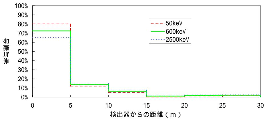
図 D.11 in-situ 測定における周囲からの寄与割合 ( \beta : 4.8 g/cm 2 )
