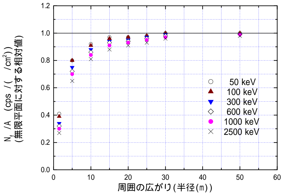
図 D.5 周囲の広がりによる計測値への影響 (検出器：p型 4.8\text{g/cm}^2 )
