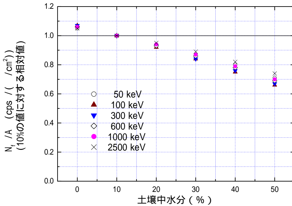
図 D.16 土壤中水分による計測値への影響 (放射性物質が土壤中に浸透した場合、 \rho : 4.8g/cm 2 )
