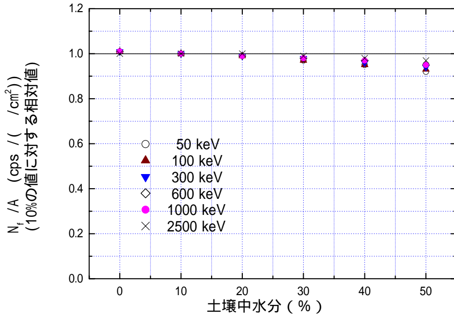
図 D.15 土壤中水分による計測値への影響 (放射性物質が地表近くに分布している場合、 \rho : 0.1g/cm 2 )
