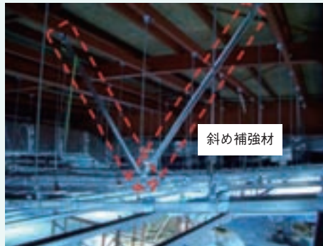
斜め補強材 金属下地天井の更新に伴う補強 「学校施設の非構造部材の耐震対策事例集」より
