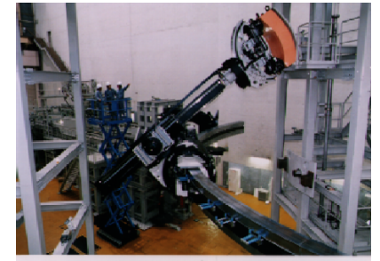
遠隔保守機器 (日,欧)
