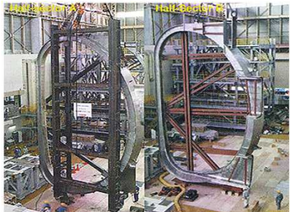
真空容器 (欧,韓,印,露)
