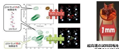
アミロイドタンパク質の二次構造を決定する新手法の開発
