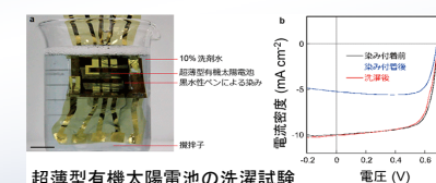
超薄型有機太陽電池の洗濯試験
