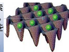
光格子の模式図
